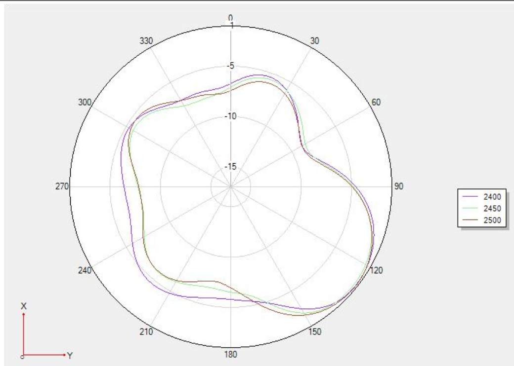
Theta 90° 方向 图
