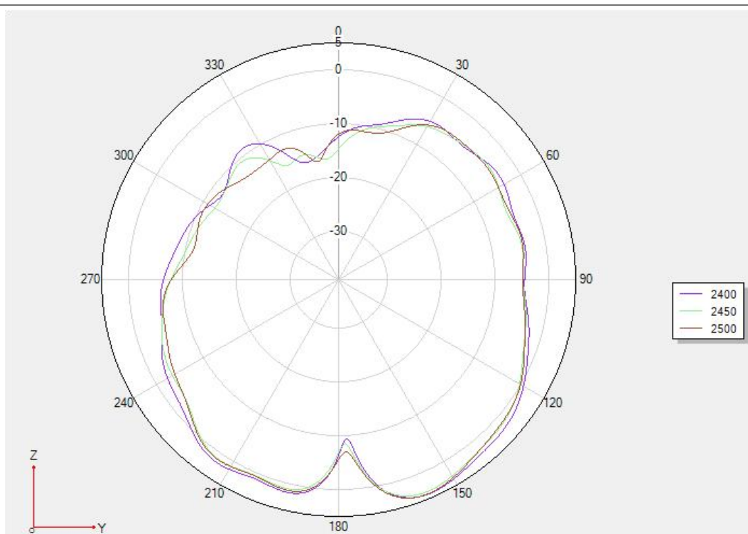
PHi 90° 方向图
