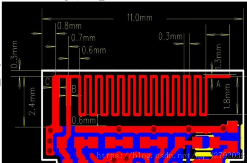
图 Nano Dongle PIFA 天线
