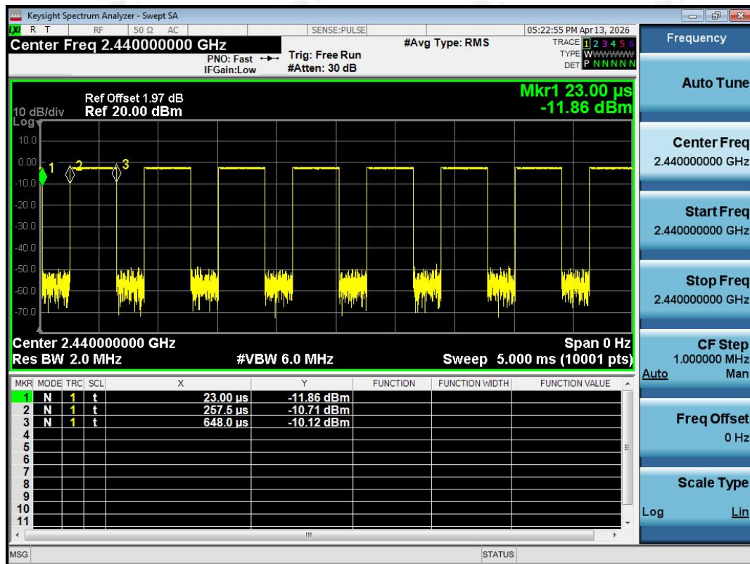
Duty Cycle NVNT BLE 1M 2440MHz Ant1
