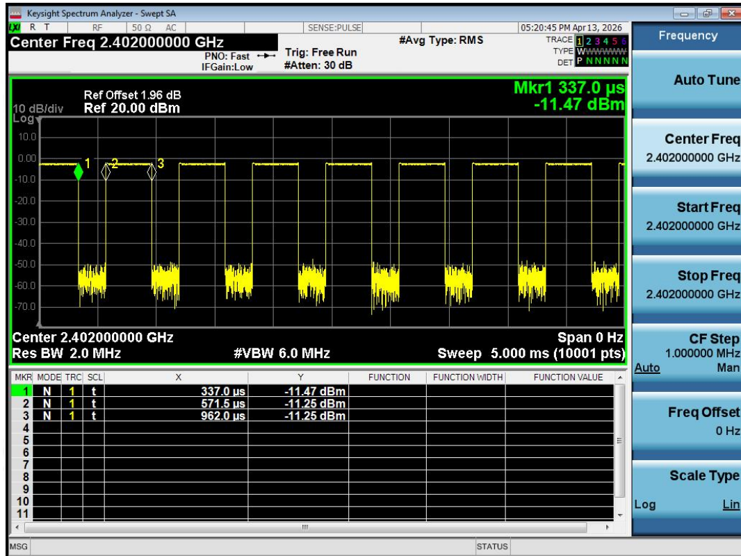
Duty Cycle NVNT BLE 1M 2402MHz Ant1
