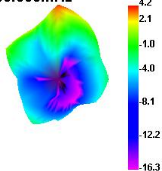
5500.000MHz
