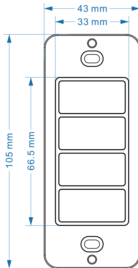
正面
