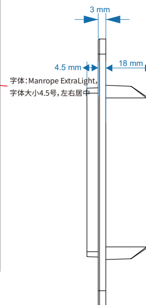
側面
