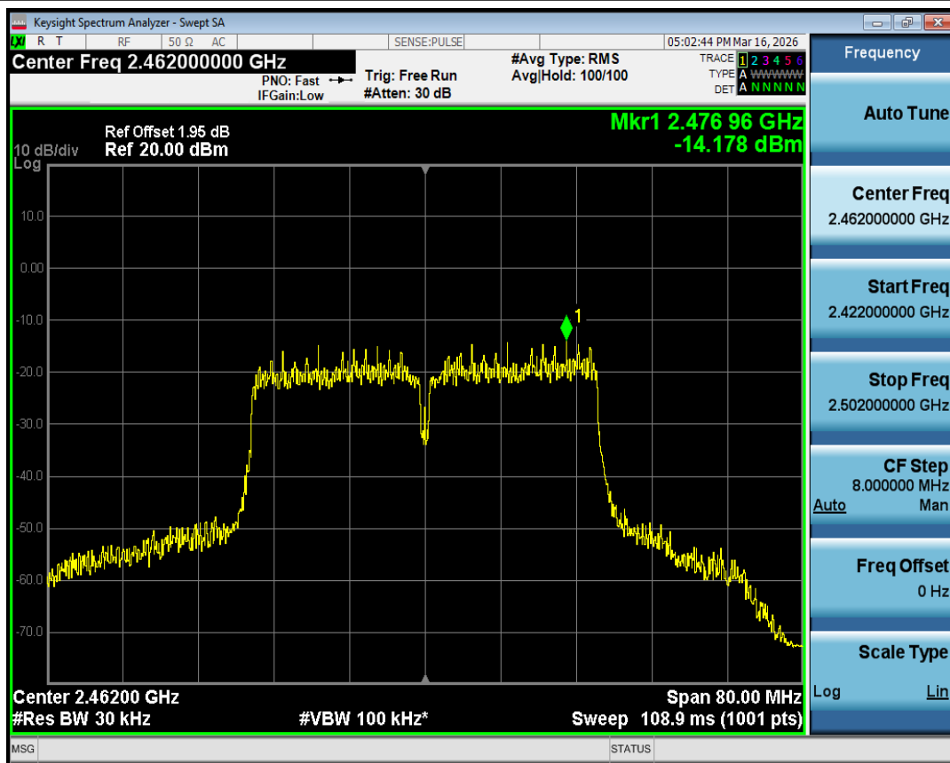
PSD NVNT n40 2462MHz Ant1
