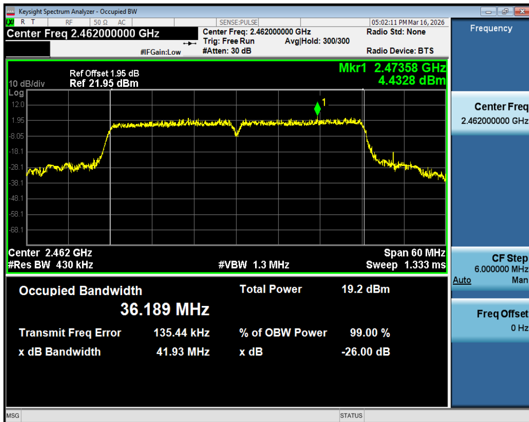
OBW NVNT n40 2462MHz Ant1
