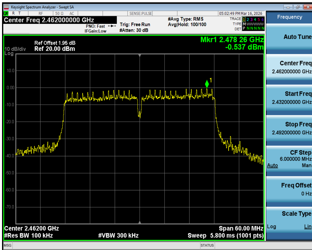
Band Edge NVNT n40 2462MHz Ant1 Ref
