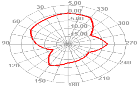
2400.000MHz E1
