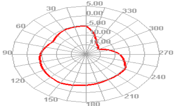
5800.000MHz H
