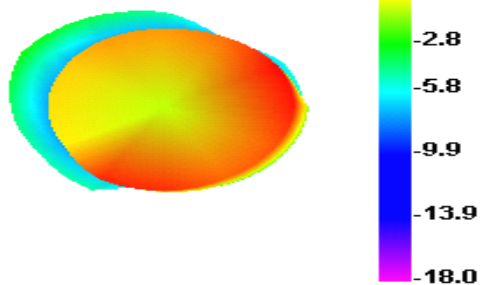
5800.000MHz E1
