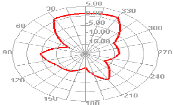
5800.000MHz E2
