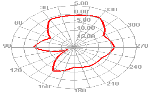
2400.000MHz E2
