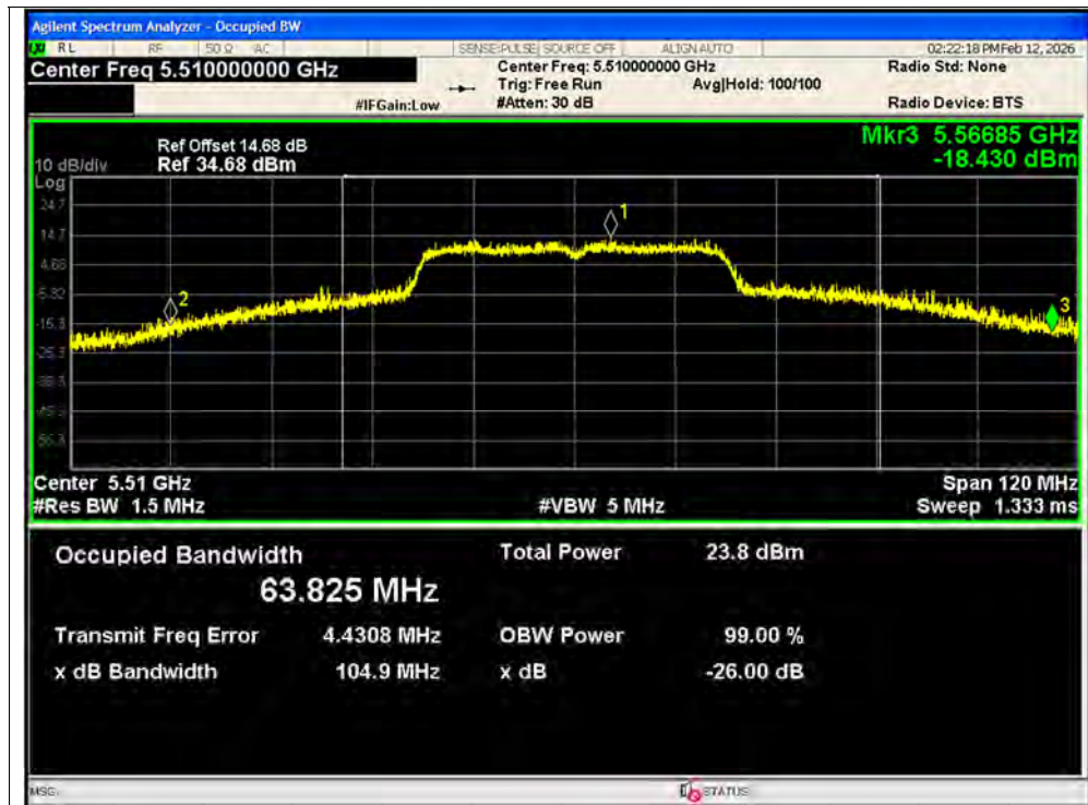
-26dB Bandwidth NVNT n40 5510MHz Ant1
