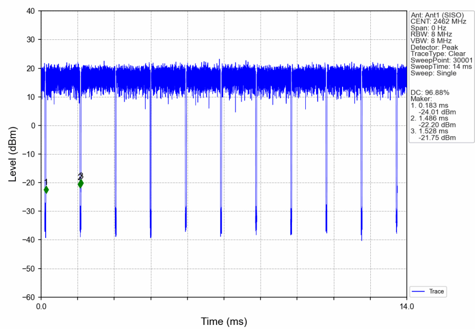
802.11n(HT20)_HCH_2462MHz_Ant1 (SISO)_NTNV
