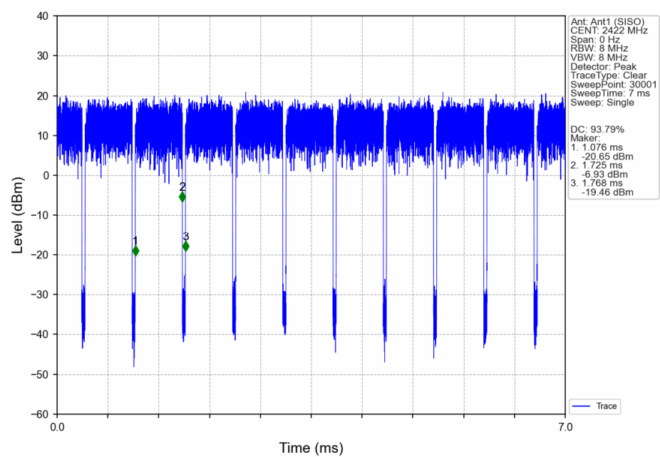
802.11n(HT40)_LCH_2422MHz_Ant1 (SISO)_NTNV
