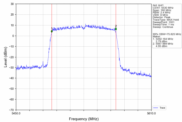
802.11ac(VHT80) U-NII-2C Low channel
