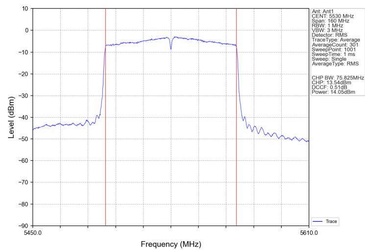
802.11ac(VHT80) U-NII-2C Low channel
