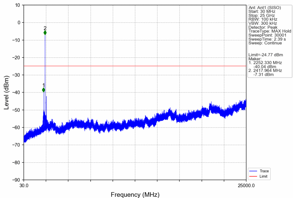
802.11ax(HEW20)_LCH_2412MHz_SU_/_Ant1 (SISO)_NTNV
