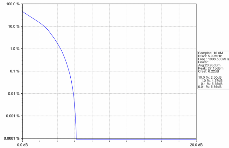
Band2 3MHz QPSK HCH 1908.5MHz RB 15 0 NTV
