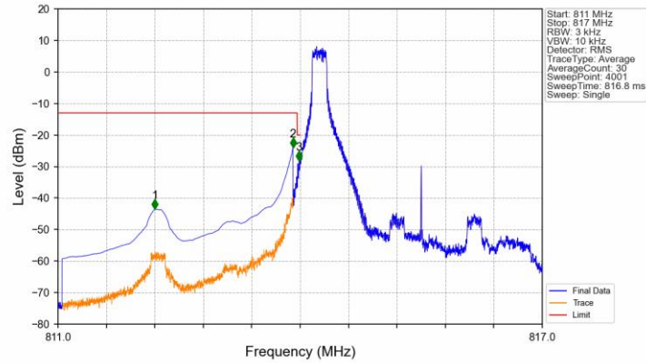
Band26a 3MHz QPSK LCH 815.5MHz RB 1 0 NTV
