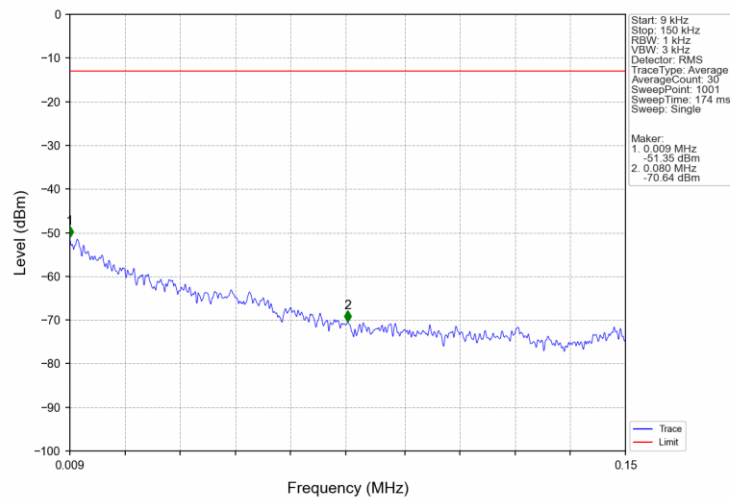
Band26a 5MHz QPSK LCH 816.5MHz RB 1 0 NTV
