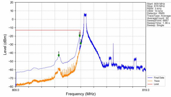
Band26a 5MHz QPSK LCH 816.5MHz RB 1 0 NTV
