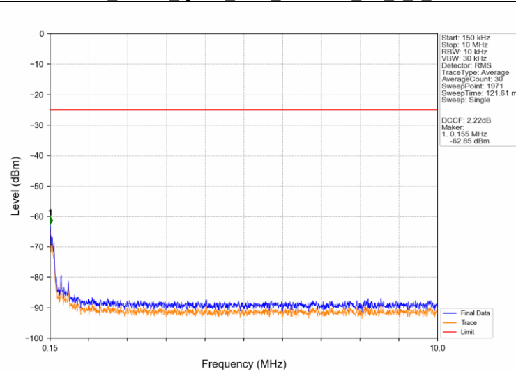
Band41_20MHz_QPSK_HCH_2645MHz_RB_1_0_NTNV
