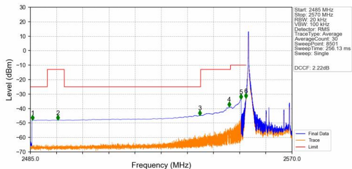
Band41_15MHz_QPSK_LCH_2562.5MHz_RB_1_0_NTNV
