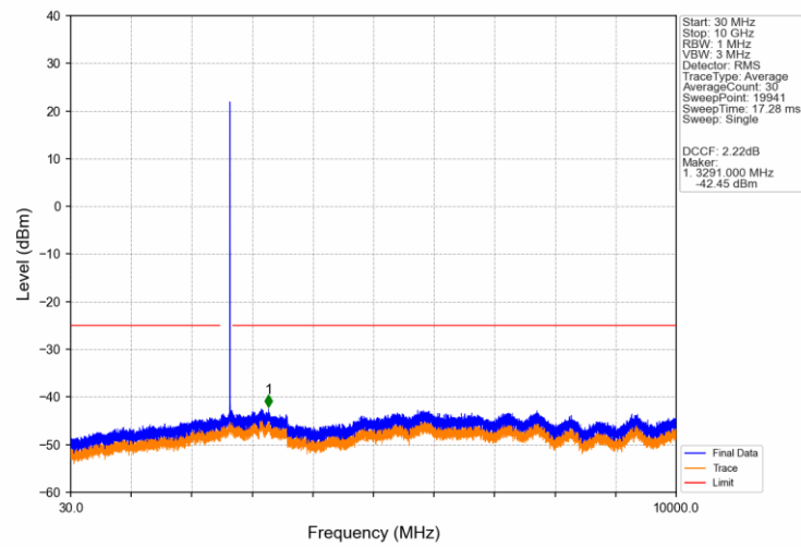
Band41_5MHz_QPSK_HCH_2652.5MHz_RB_1_0_NTNV
