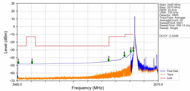
Band41_15MHz_QPSK_LCH_2562.5MHz_RB_1_0_NTNV
