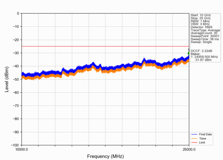
Band41_15MHz_QPSK_MCH_2605MHz_RB_1_0_NTNV
