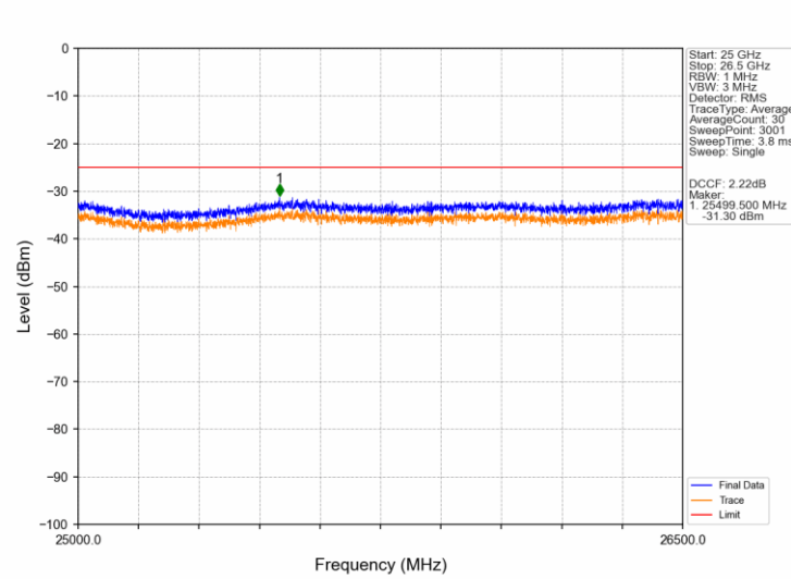
Band41_15MHz_QPSK_MCH_2605MHz_RB_1_0_NTNV
