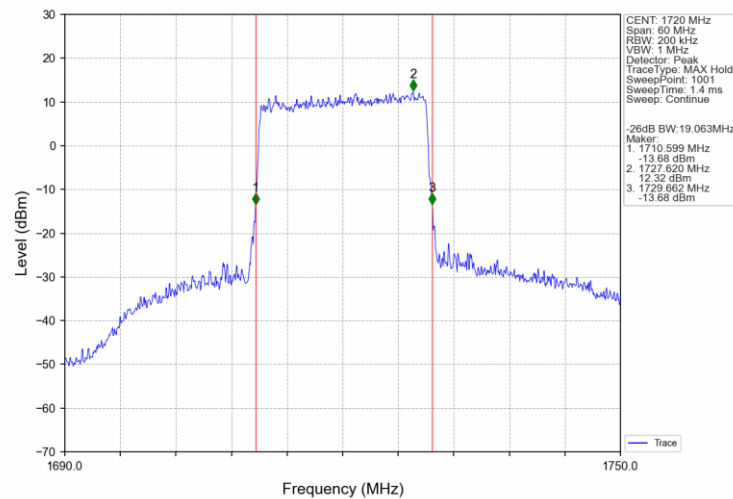
Band66 20MHz 16QAM LCH 1720MHz RB 100 0 NTNV
