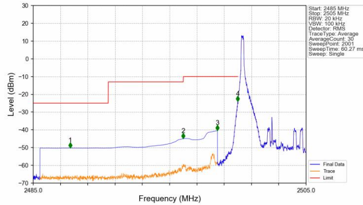
Band7_5MHz_QPSK_LCH_2502.5MHz_RB_1_0_NTNV
