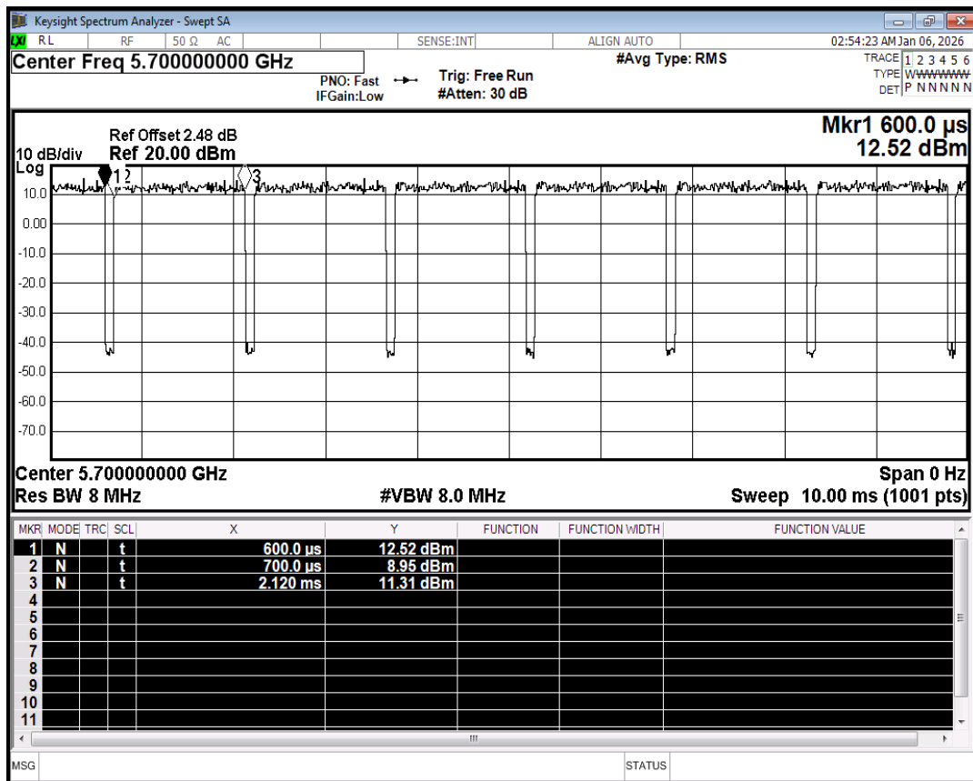
Duty Cycle NVNT a 5700MHz Ant1
