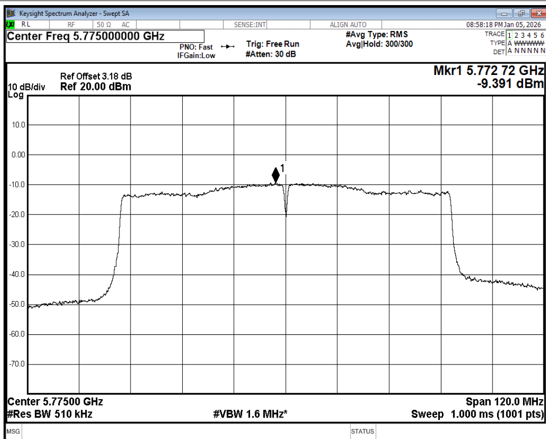
PSD NVNT ac80 5775MHz Ant1
