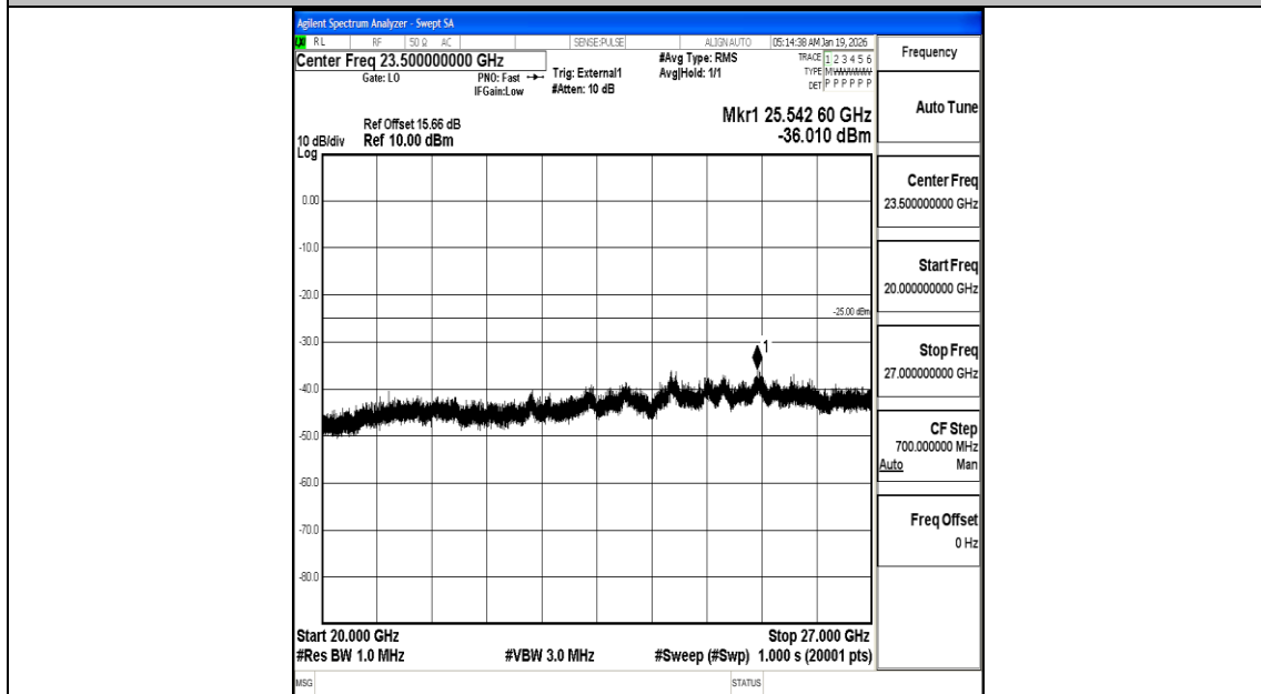
Band38_ 15MHz_ 16QAM_ 37825_ 1RB#0_ 20000~27000_ 20000~27000
