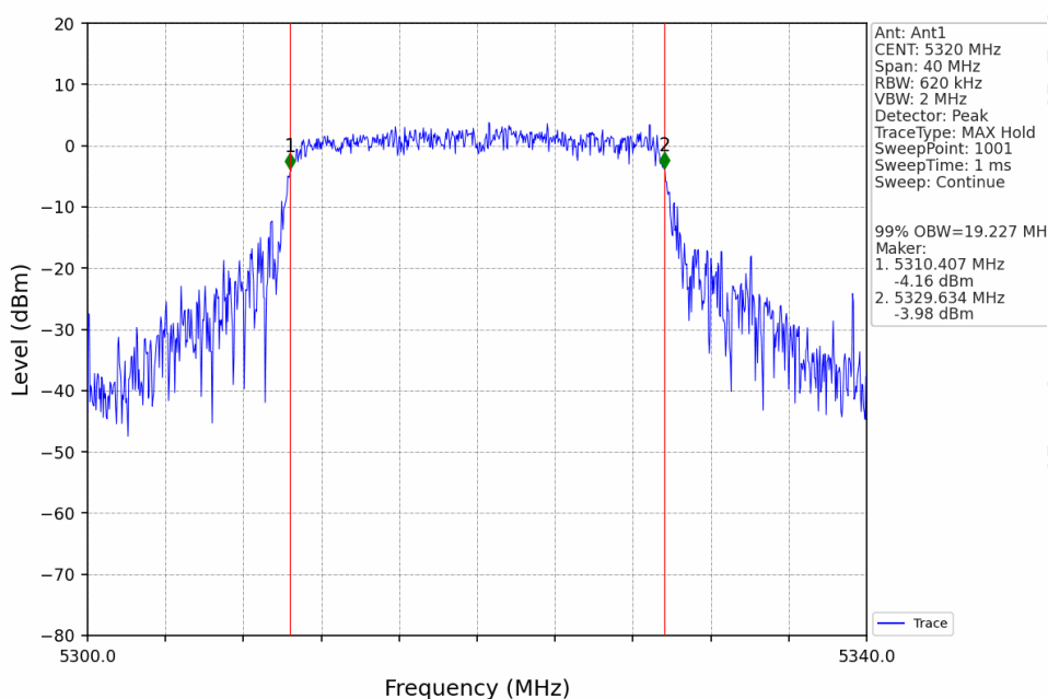
802.11ax(HEW20) HCH 5320MHz SU / Ant1 NTV
