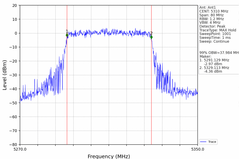
802.11ax(HEW40) HCH 5310MHz SU / Ant1 NTV
