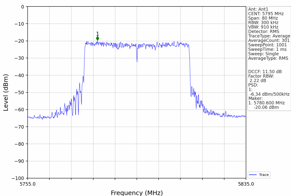
802.11ax(HEW40) HCH 5795MHz SU / Ant1 NTN
