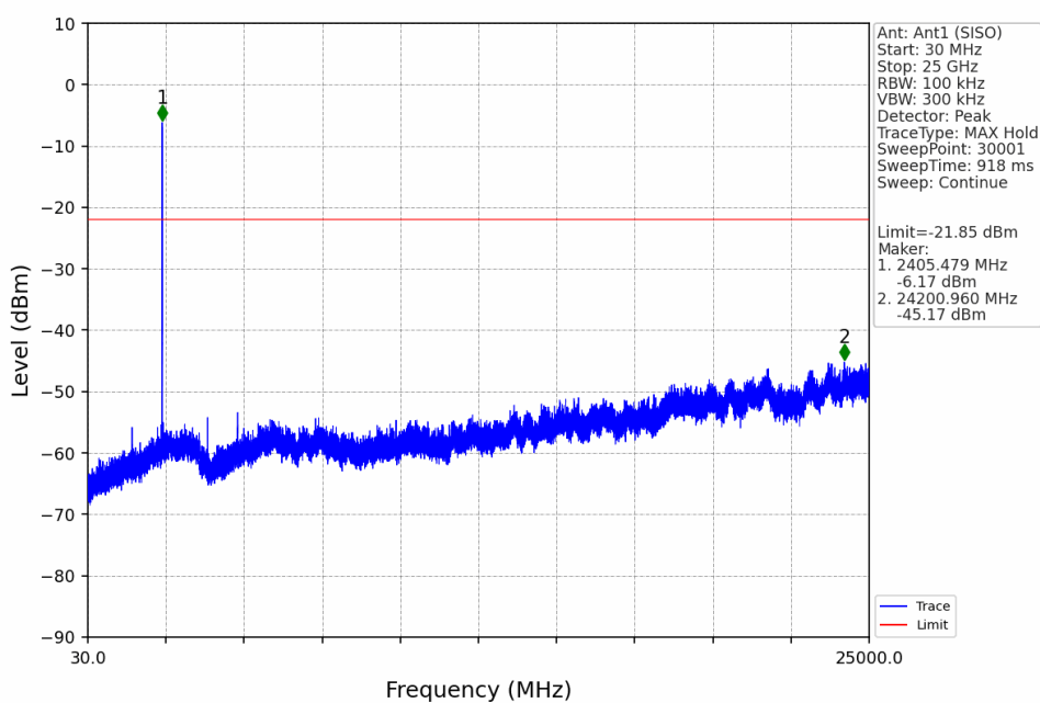
802.11ax(HEW20) LCH 2412MHz SU / Ant1 (SISO) NTVN
