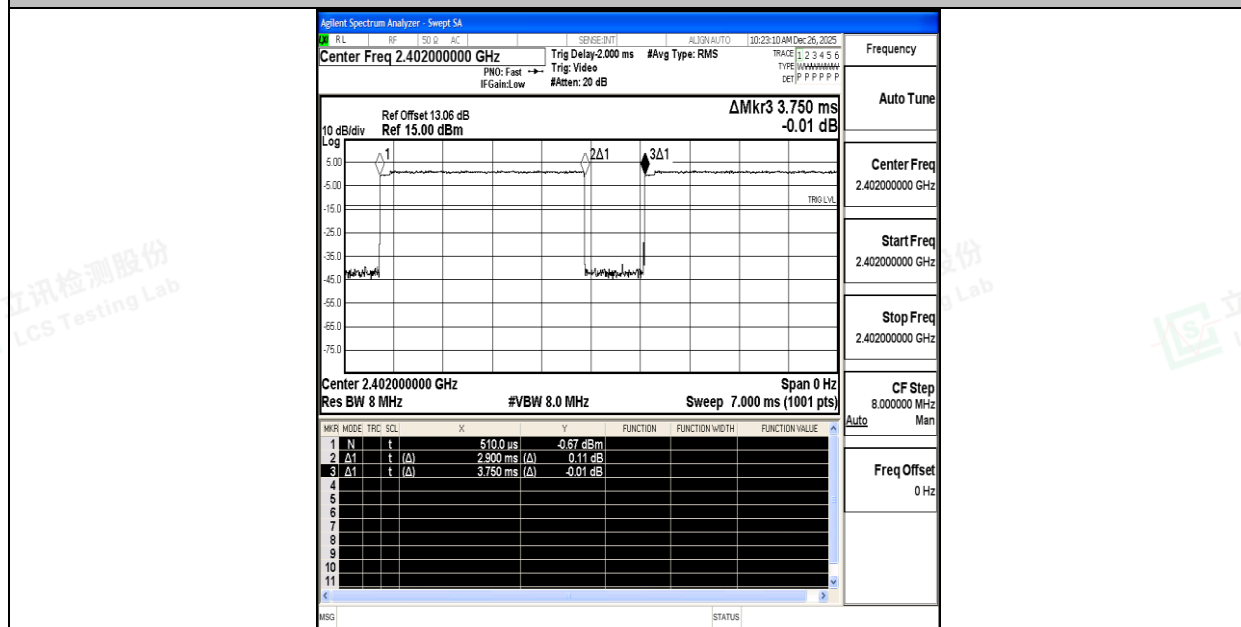
NTNV-2DH5-Ant1-2402
