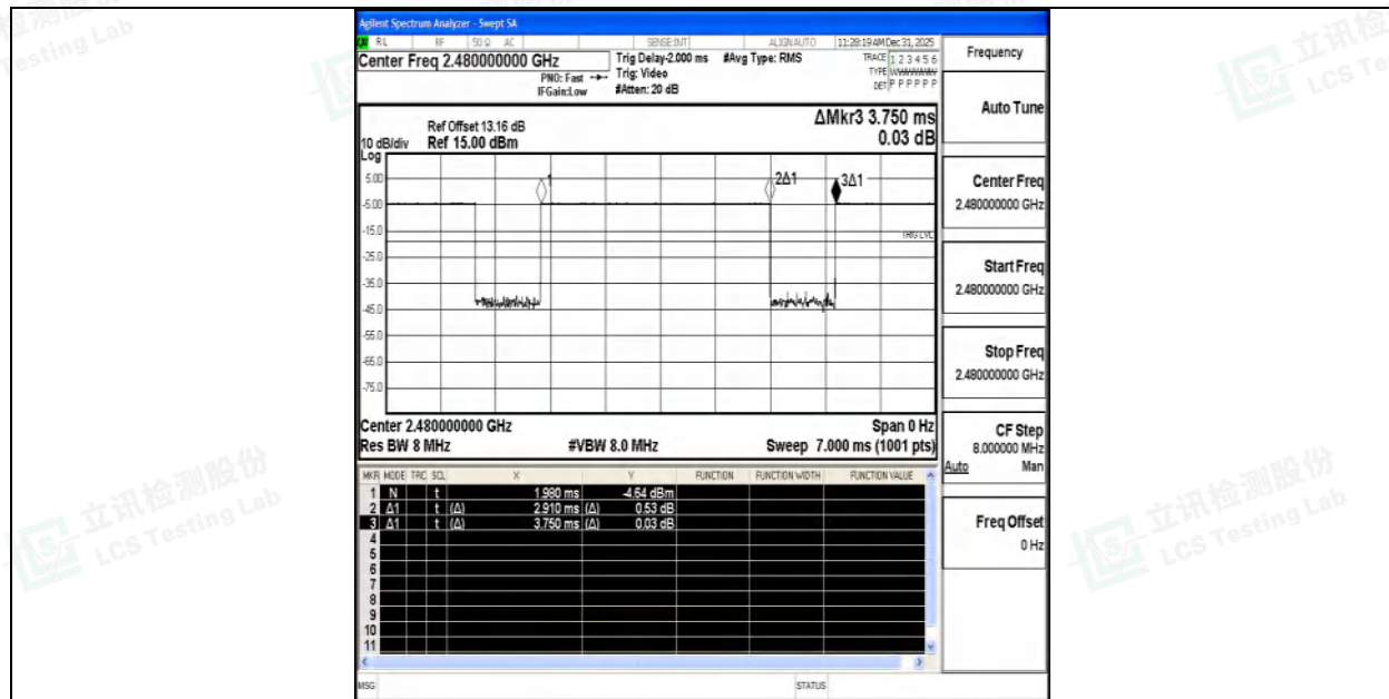
NTNV-DH5-Ant1-2480
