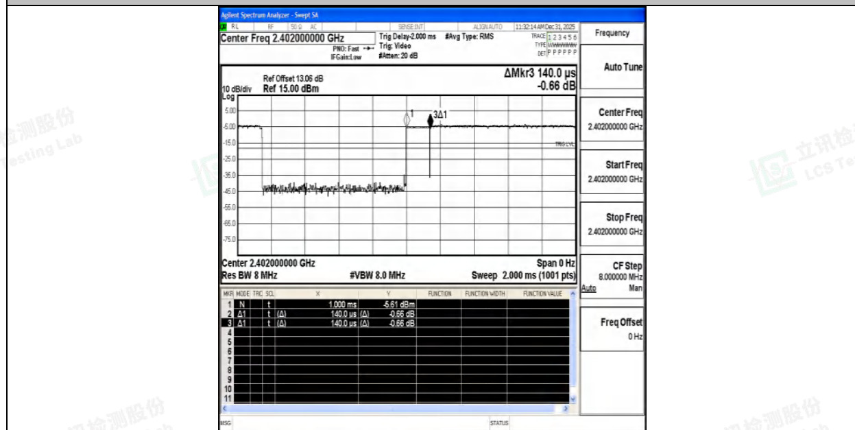
NTNV-2DH5-Ant1-2402
