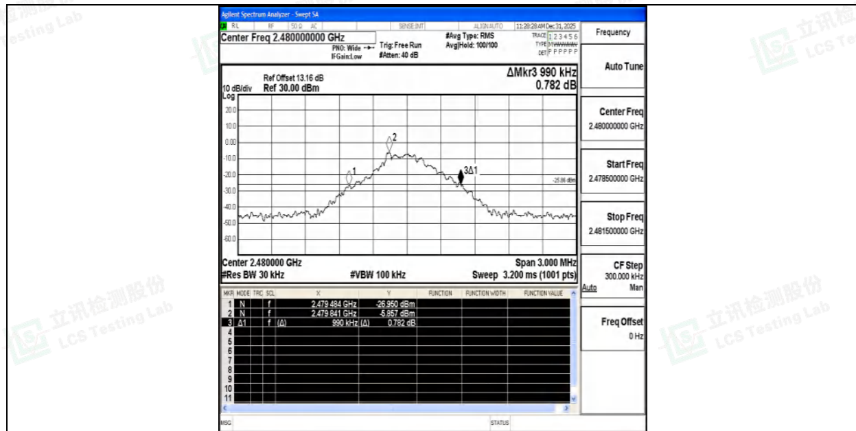
DH5-Ant1-2480
