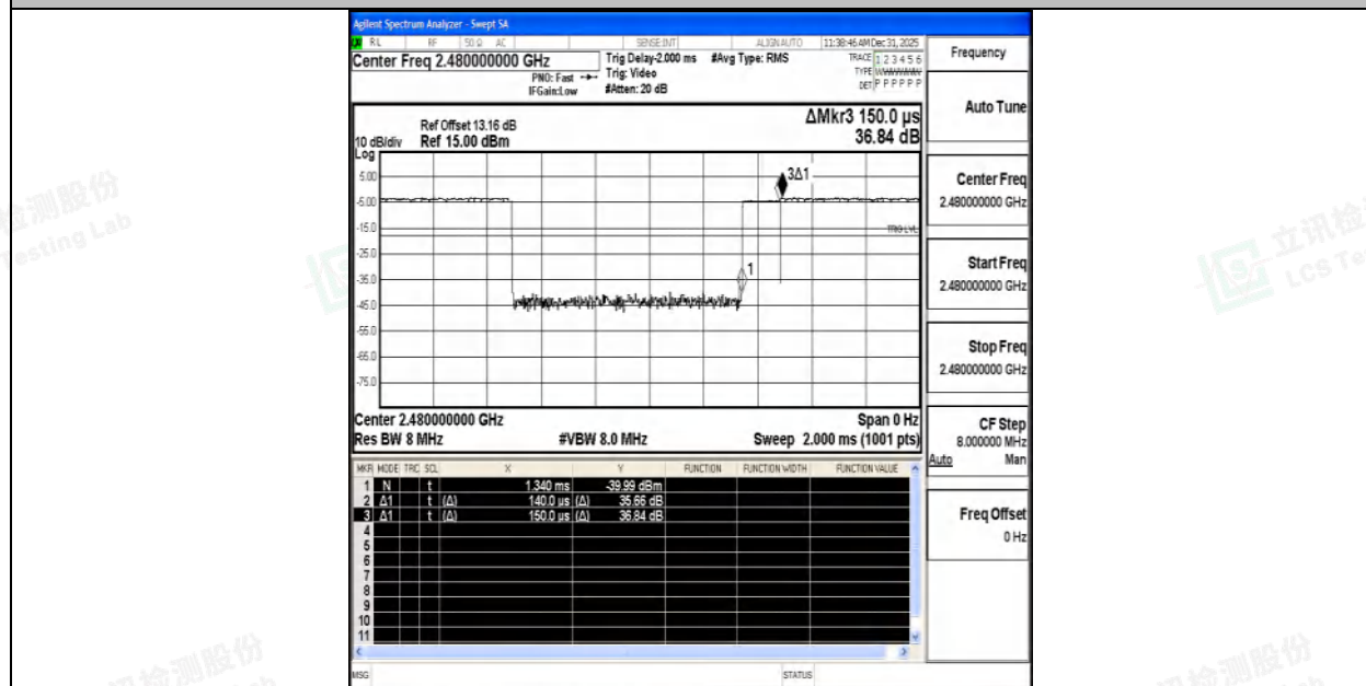
NTNV-2DH5-Ant1-2480
