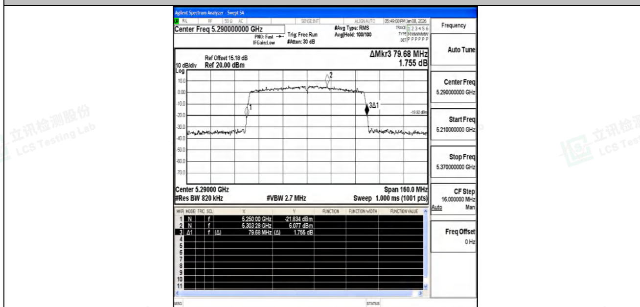
11AC80SISO-Ant1-5290
