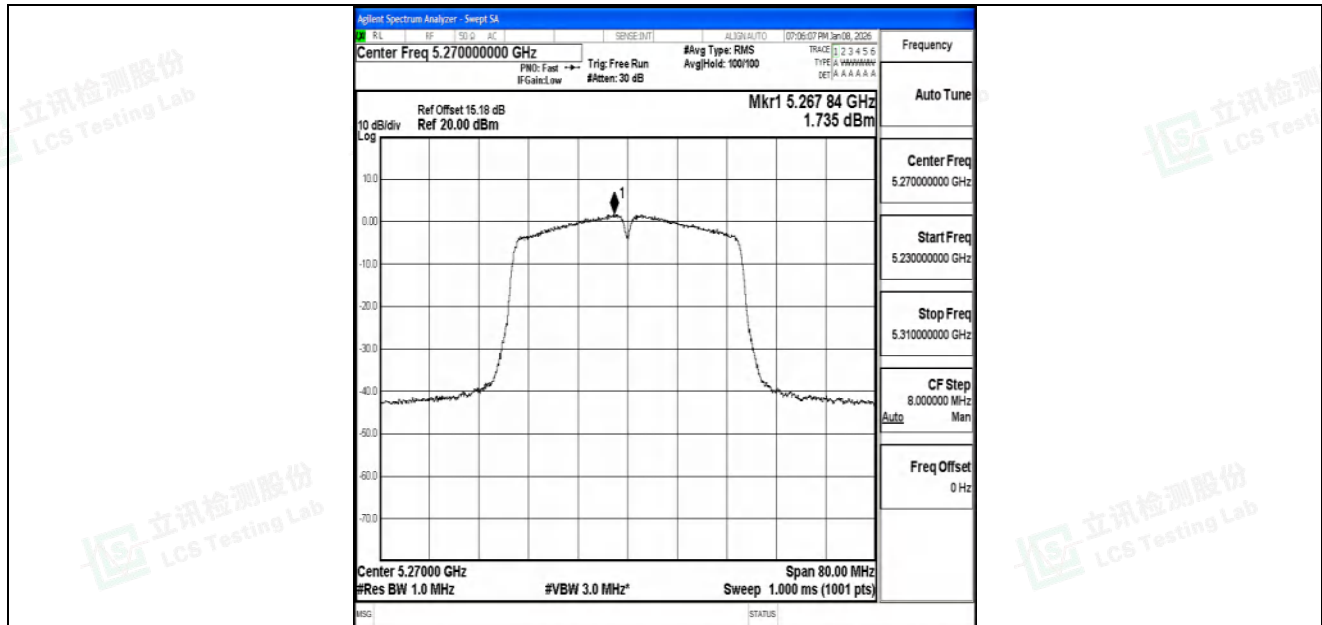
11N40SISO-Ant2-5270-PASS
