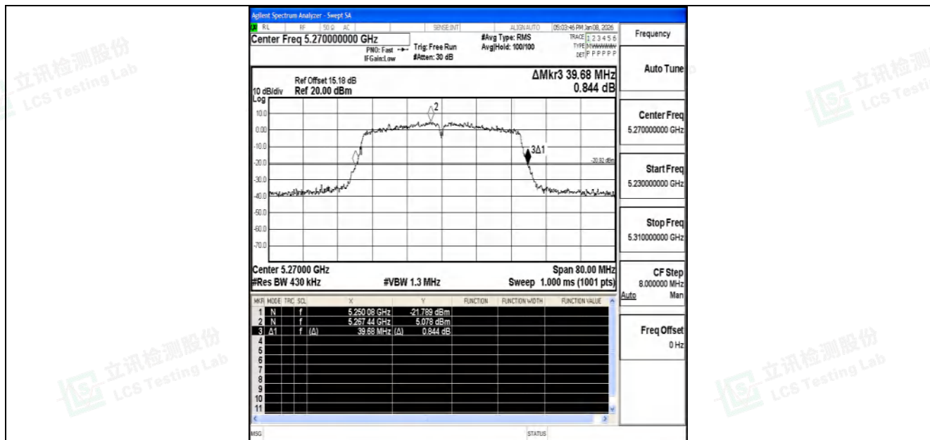
11N40SISO-Ant1-5270
