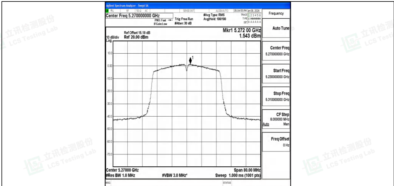
11N40SISO-Ant1-5270-PASS
