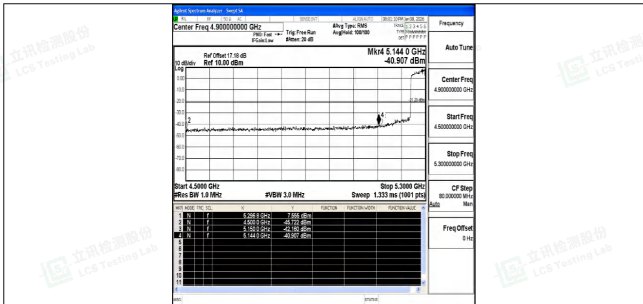
11AC80SISO-Ant2-5290-PASS
