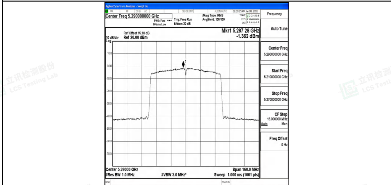
11AC80SISO-Ant2-5290-PASS
