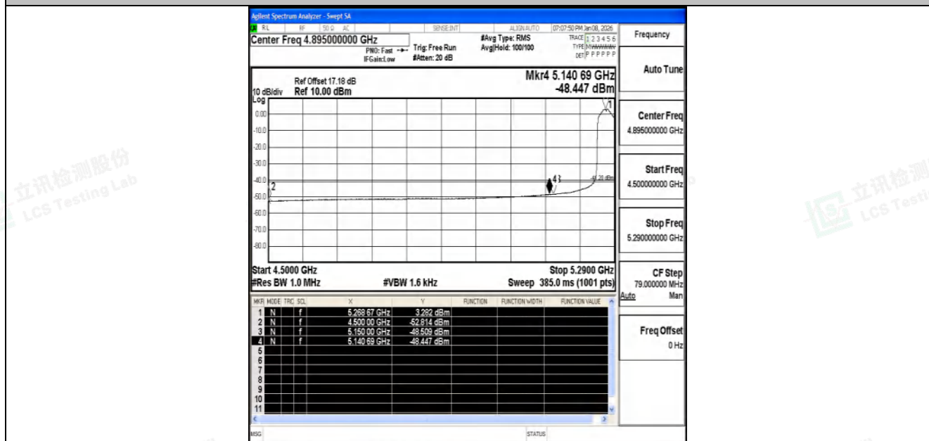
11N40SISO-Ant2-5270-PASS
