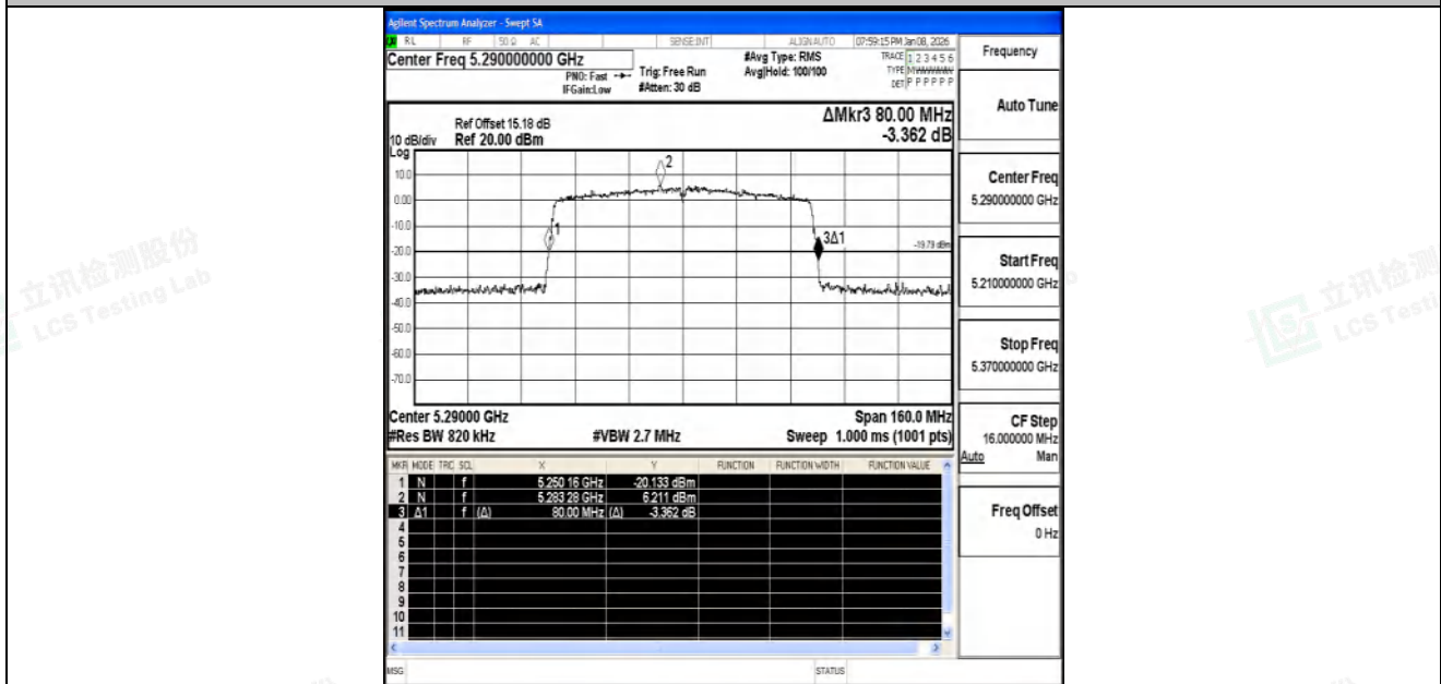
11AC80SISO-Ant2-5290
