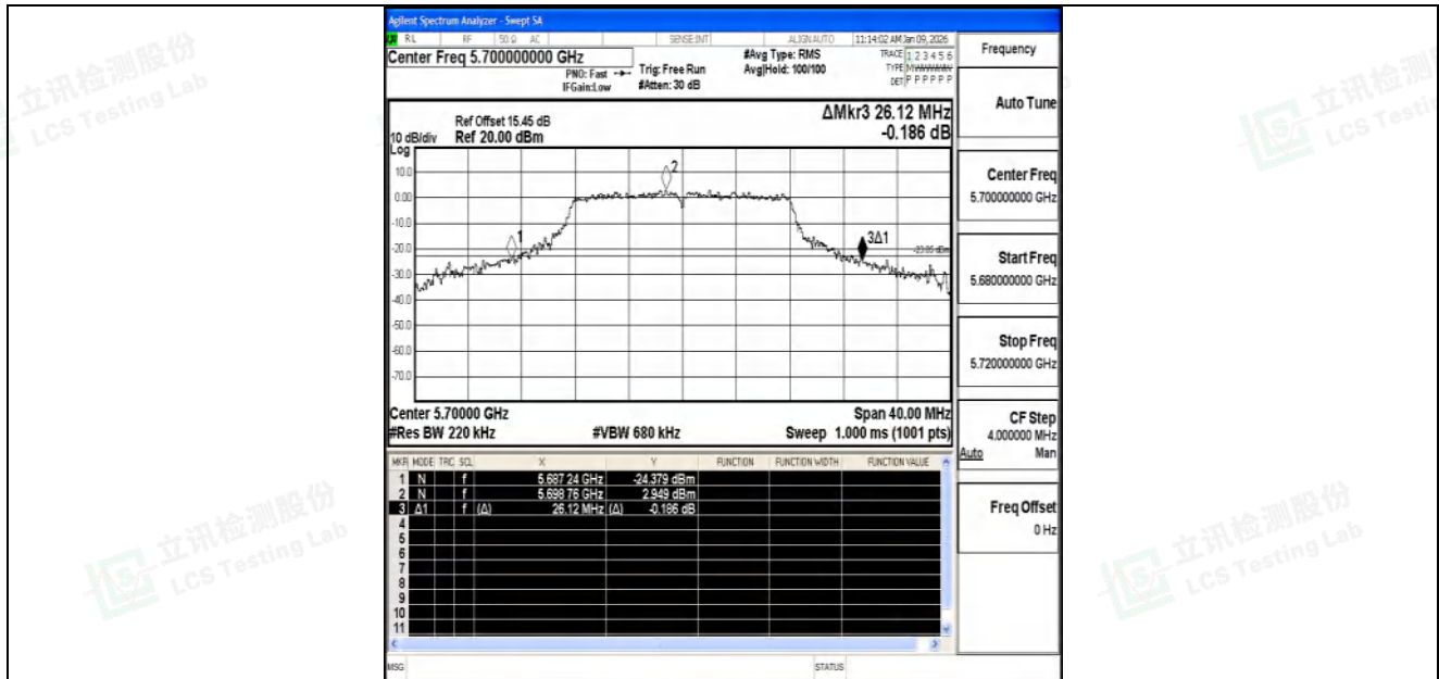
11A-Ant1-5700
