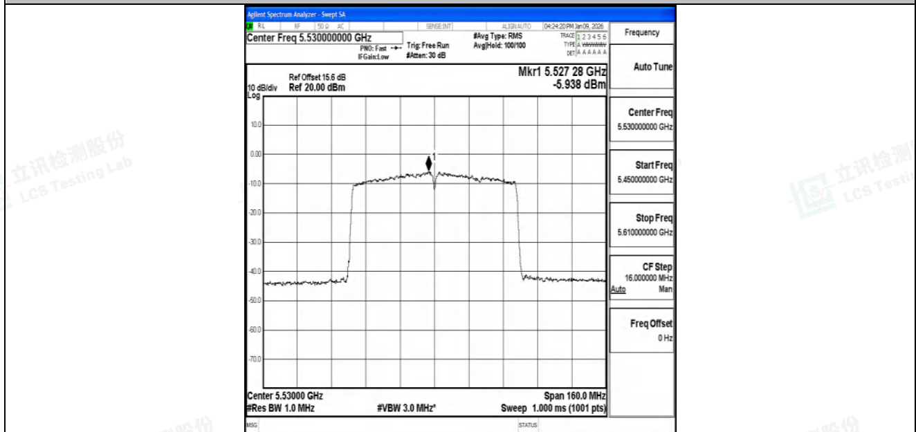
11AC80SISO-Ant2-5530-PASS
