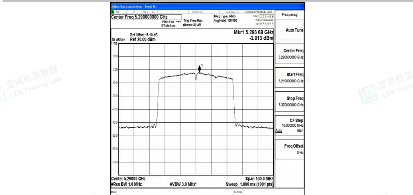
11AC80SISO-Ant2-5290-PASS
