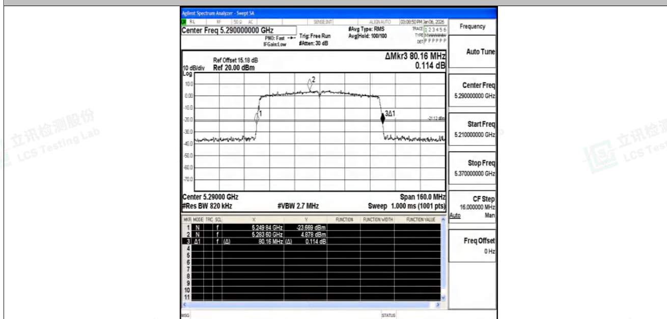
11AC80SISO-Ant2-5290
