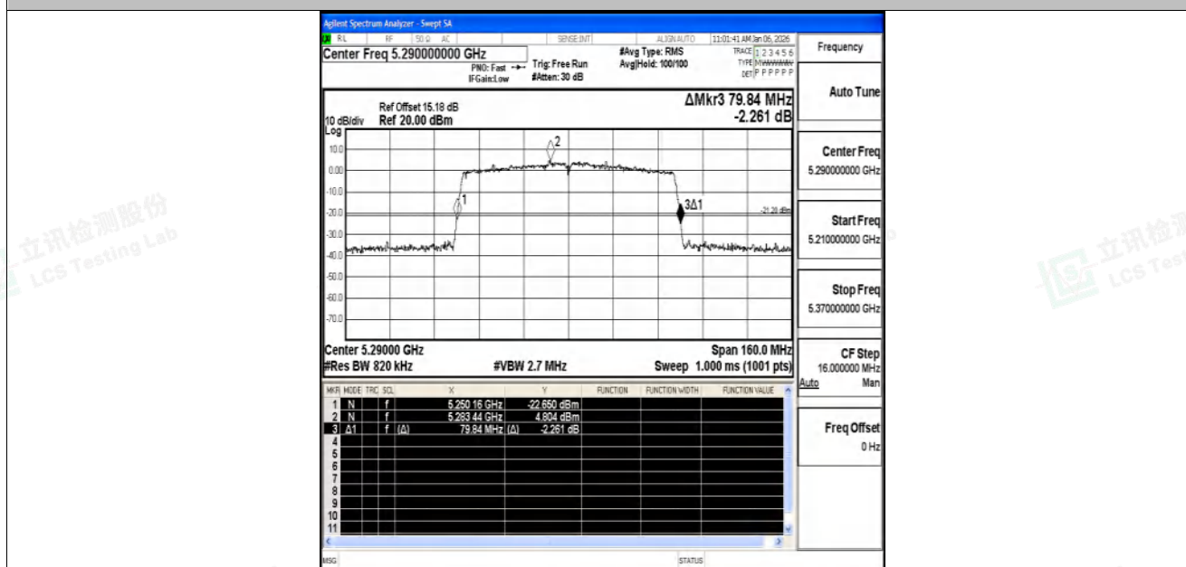
11AC80SISO-Ant1-5290
