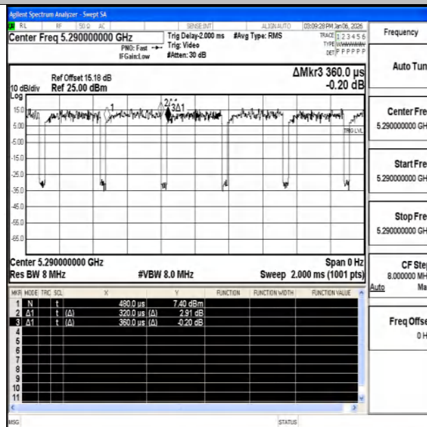
NTNV-11AC80SISO-Ant2-5290
