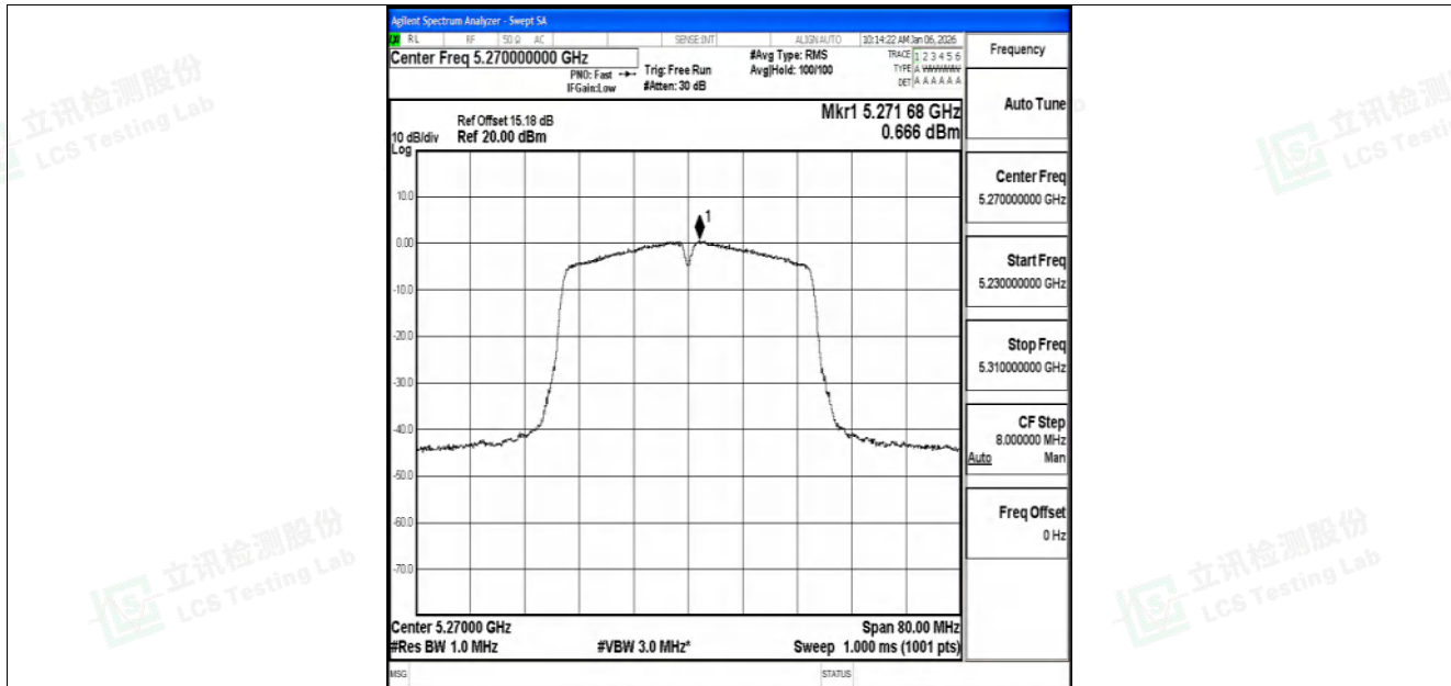
11N40SISO-Ant1-5270-PASS
