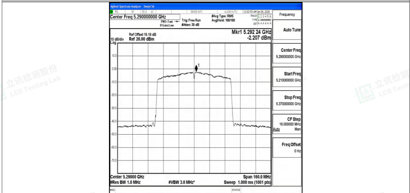
11AC80SISO-Ant1-5290-PASS
