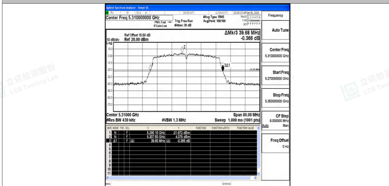
11N40SISO-Ant1-5310
