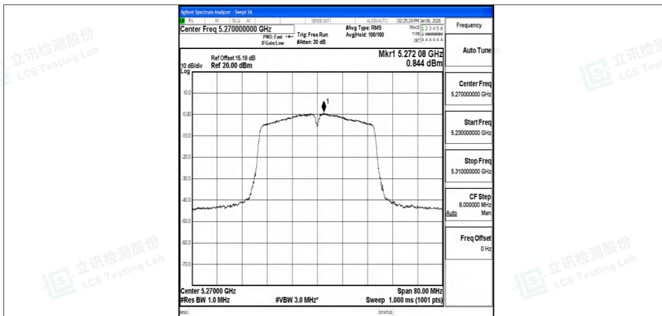
11N40SISO-Ant2-5270-PASS
