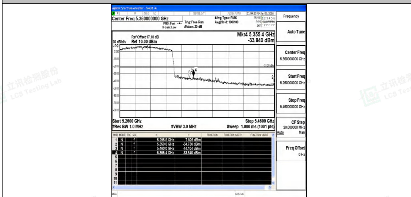
11AC80SISO-Ant1-5290-PASS
