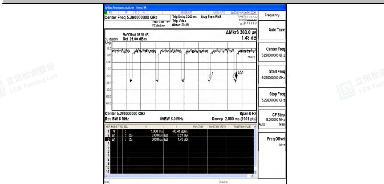
NTNV-11AC80SISO-Ant1-5290
