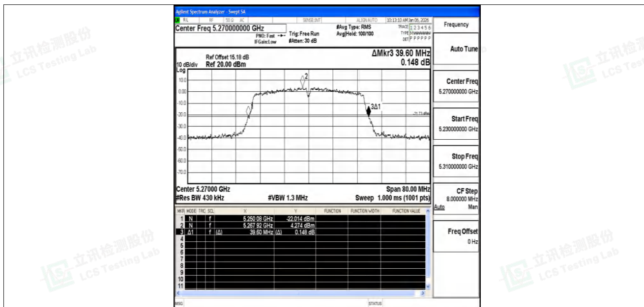
11N40SISO-Ant1-5270
