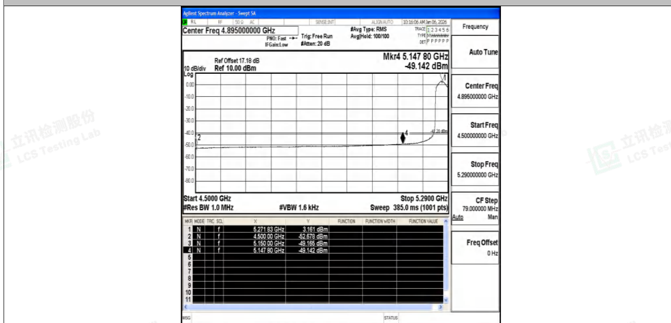
11N40SISO-Ant1-5270-PASS
