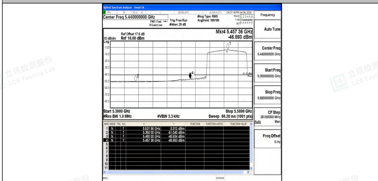
11AC80SISO-Ant1-5530-PASS
