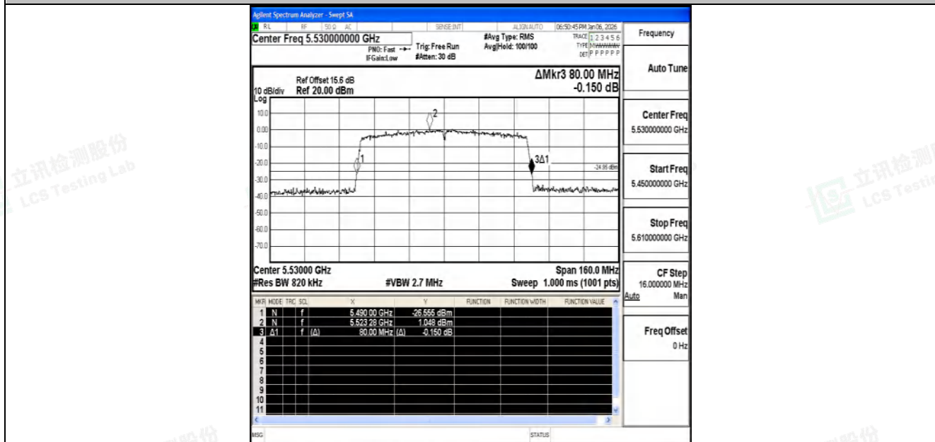
11AC80SISO-Ant2-5530
