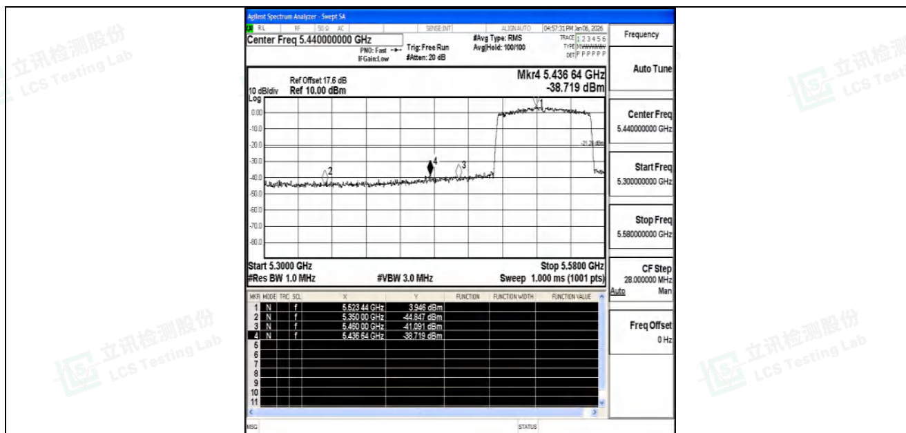
11AC80SISO-Ant1-5530-PASS
