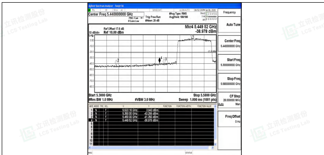
11AC80SISO-Ant2-5530-PASS
