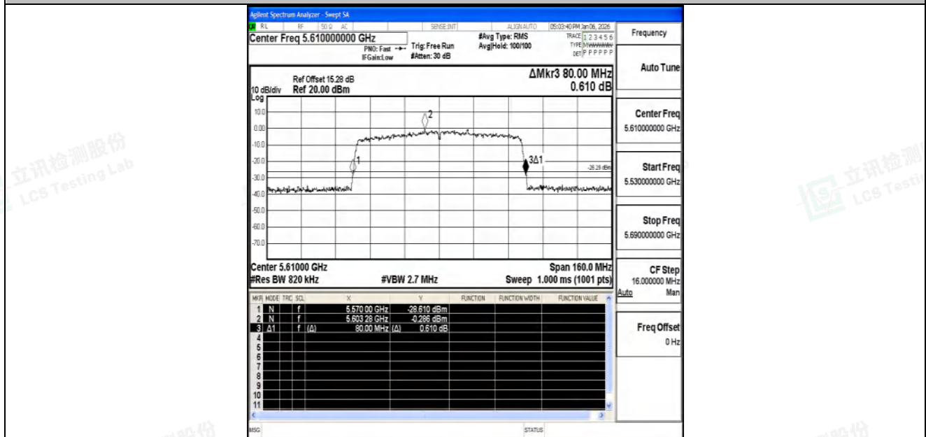
11AC80SISO-Ant1-5610
