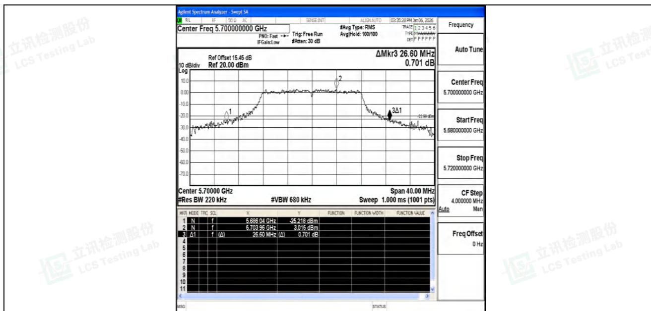
11A-Ant1-5700
