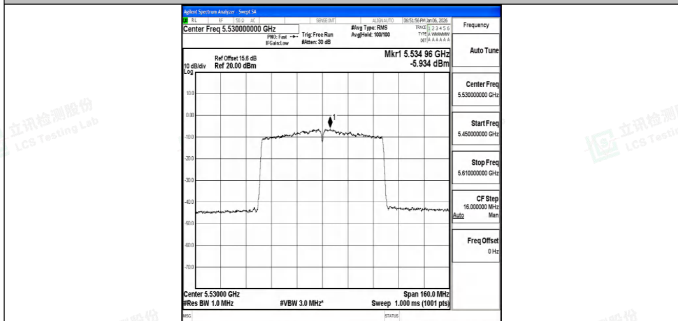
11AC80SISO-Ant2-5530-PASS
