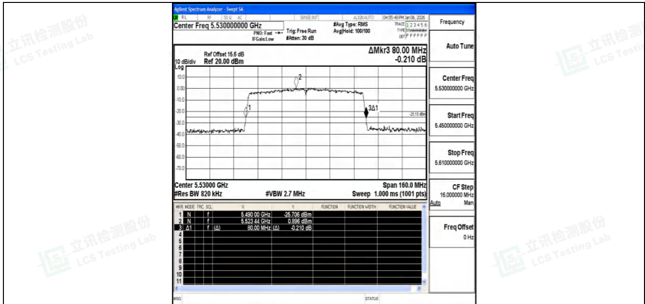
11AC80SISO-Ant1-5530
