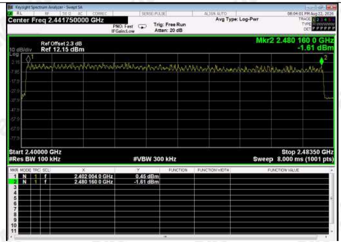
\pi/4 DQPSK Modulation
