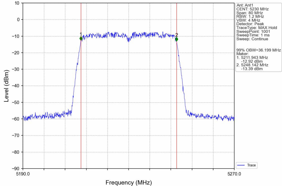
802.11ac(VHT40) HCH_5230MHz_Ant1_NTNV
