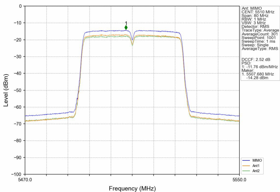
802.11ac(VHT40) LCH_5510MHz_MIMO_NTNV
