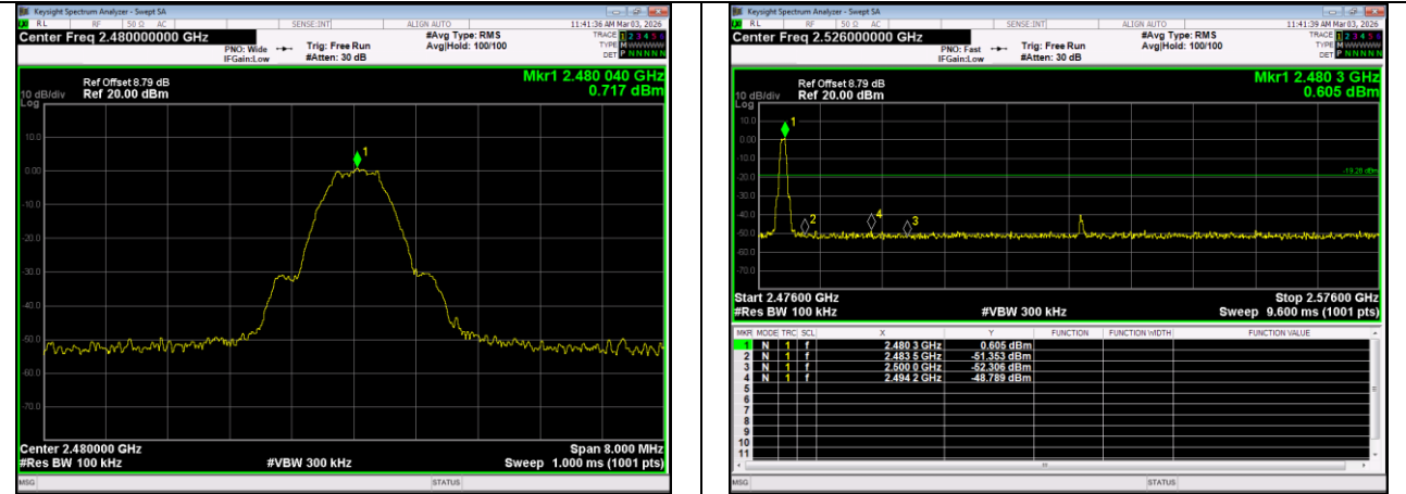
BLE 1M: Band Edge, Right Side
