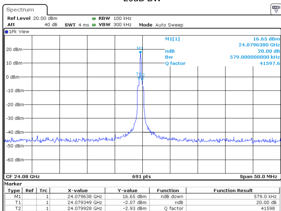
CH 01 20dB BW
