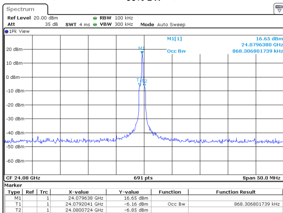
CH 01 99% BW
