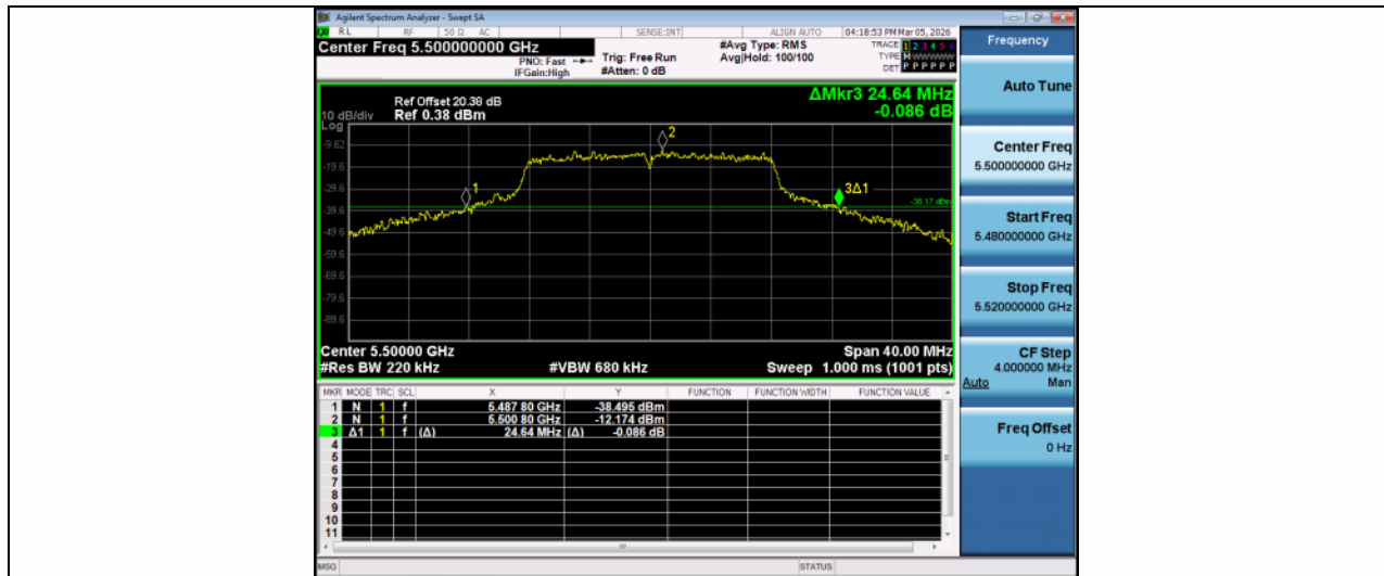
11A-Ant1-5500
