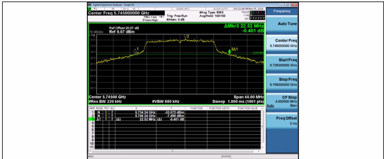
11A-Ant1-5745
