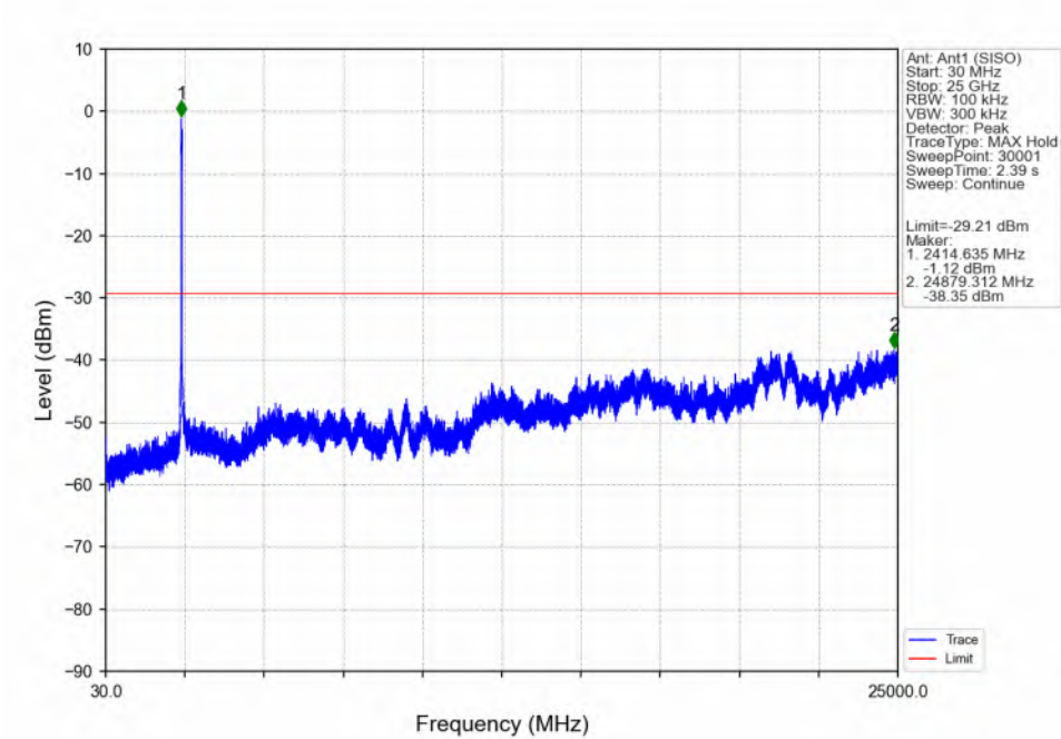
802.11n(HT40)_LCH_2422MHz_Ant1 (SISO)_NTNV
