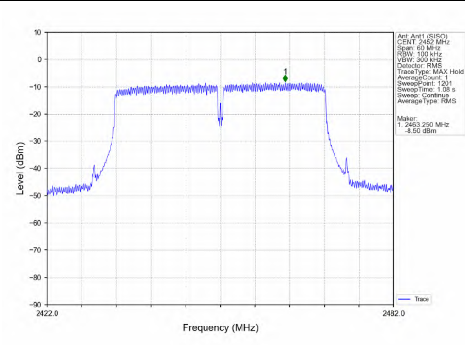
802.11n(HT40)_HCH_2452MHz_Ant1 (SISO)_NTNV
