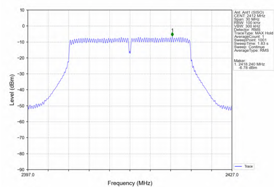
802.11n(HT20)_LCH_2412MHz_Ant1 (SISO)_NTNV
