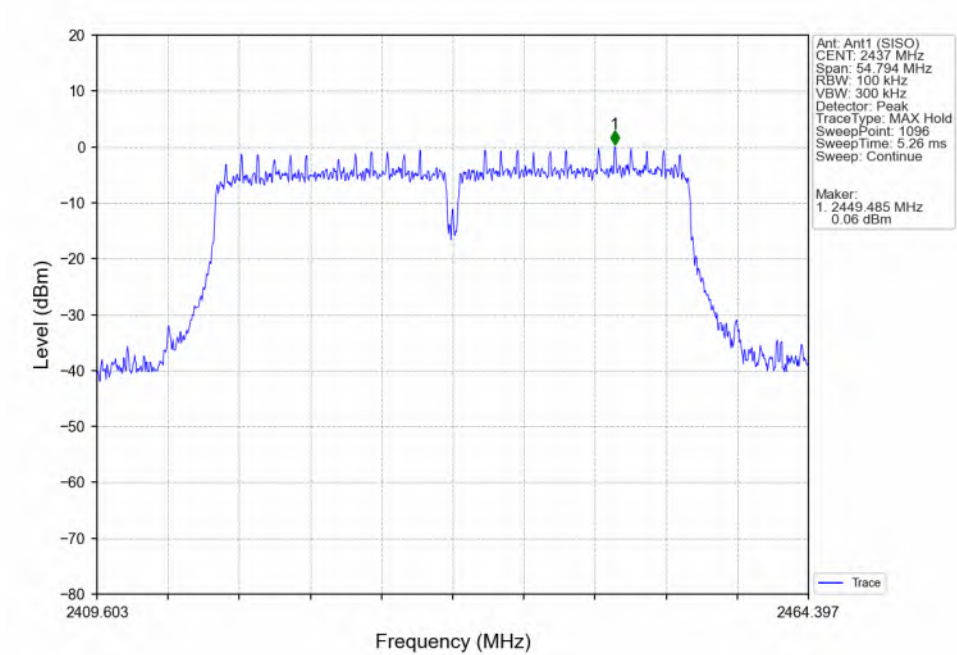
802.11n(HT40)_MCH_2437MHz_Ant1 (SISO)_NTNV
