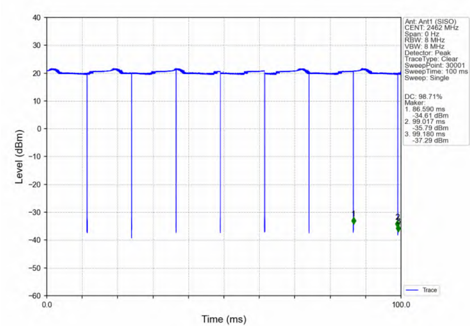
802.11b_HCH_2462MHz_Ant1 (SISO)_NTNV
