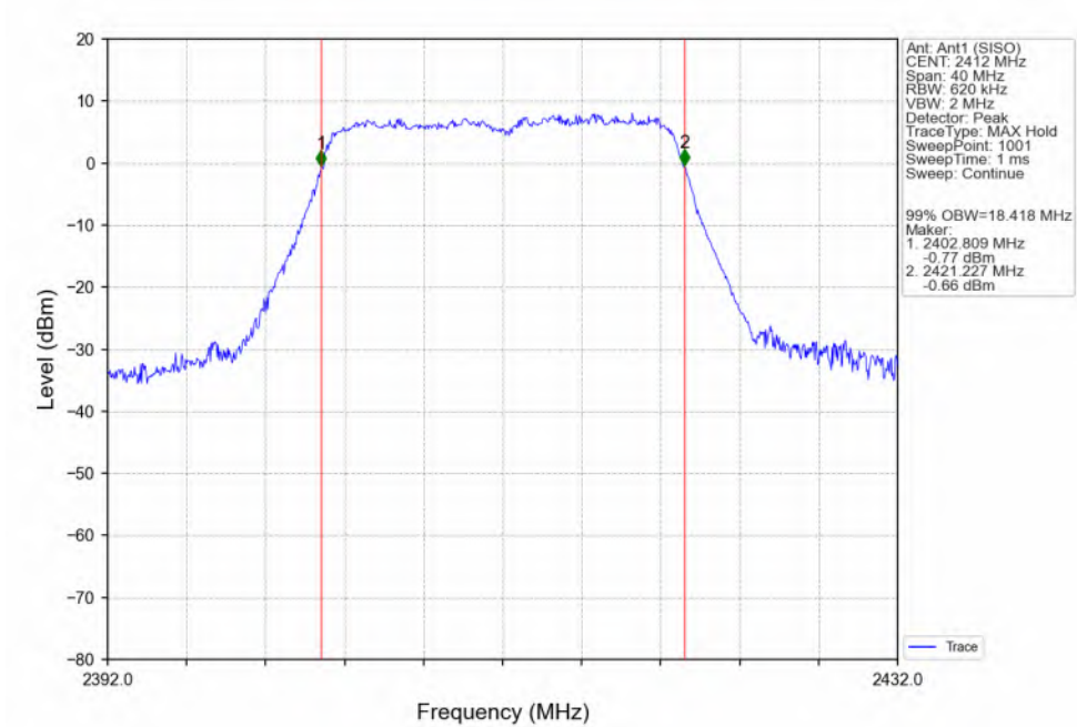
802.11n(HT20)_LCH_2412MHz_Ant1 (SISO)_NTNV
