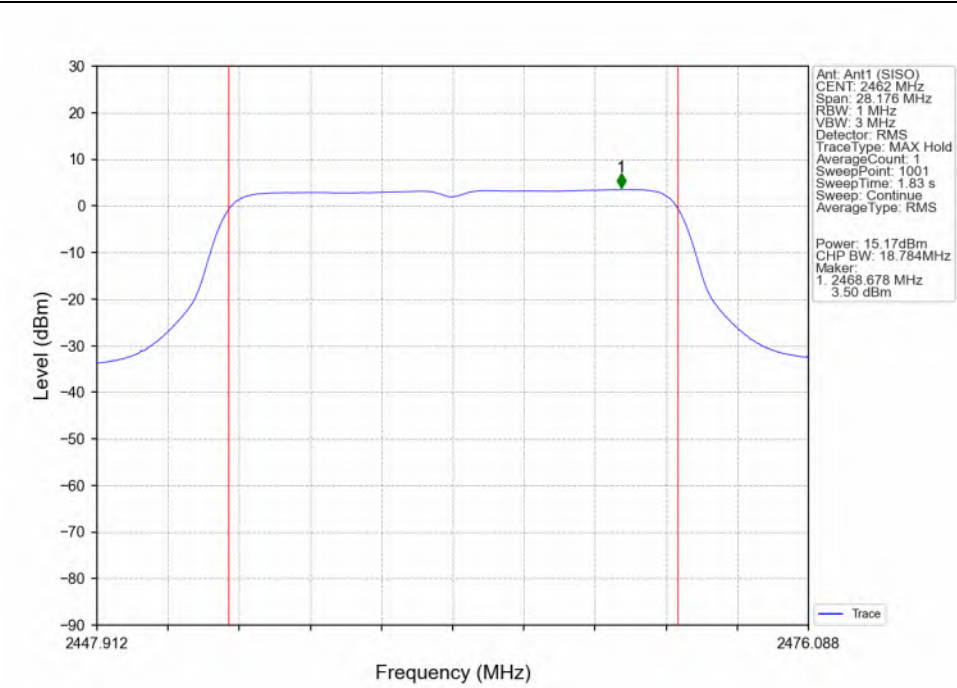
802.11n(HT20)_HCH_2462MHz_Ant1 (SISO)_NTNV
