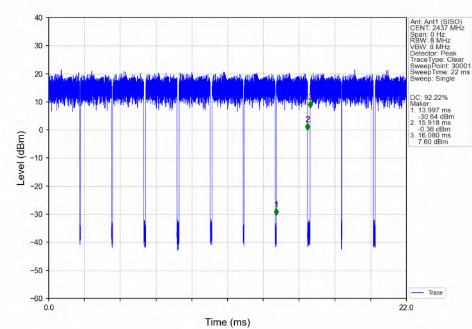
802.11n(HT20)_MCH_2437MHz_Ant1 (SISO)_NTNV
