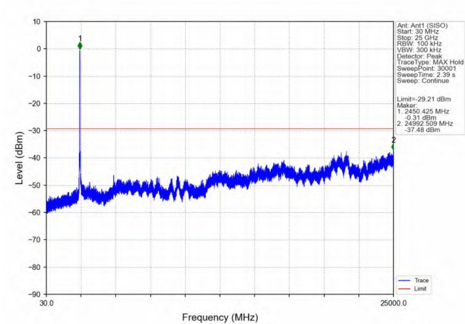
802.11n(HT40)_MCH_2437MHz_Ant1 (SISO)_NTNV
