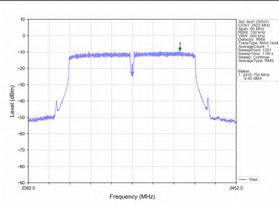
802.11n(HT40)_LCH_2422MHz_Ant1 (SISO)_NTNV
