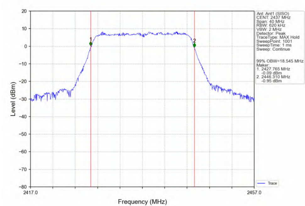
802.11n(HT20)_MCH_2437MHz_Ant1 (SISO)_NTNV
