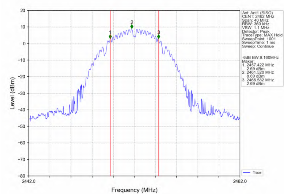
802.11b_HCH_2462MHz_Ant1 (SISO)_NTNV
