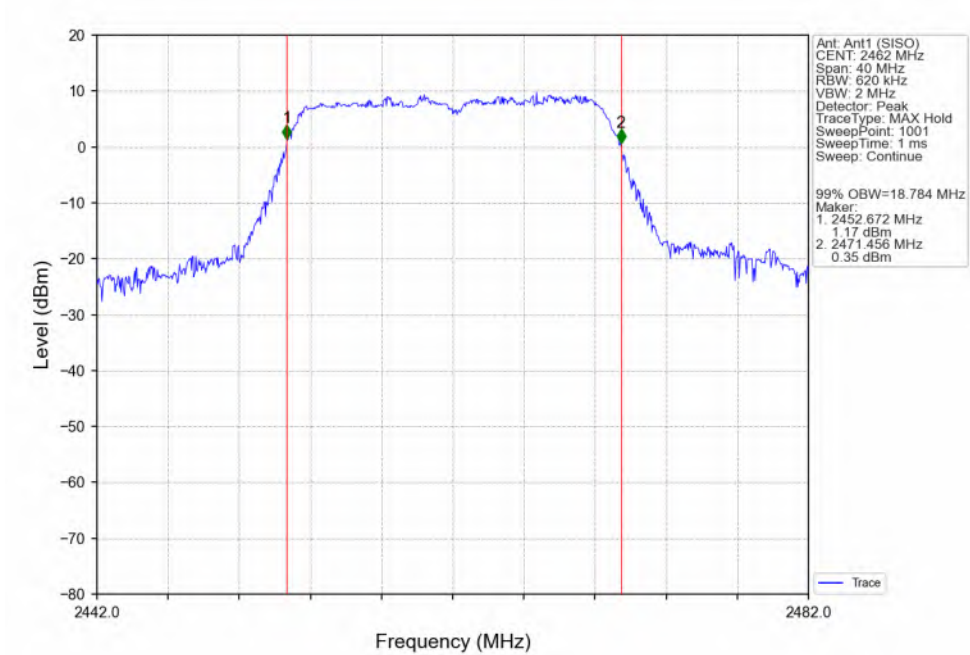
802.11n(HT20)_HCH_2462MHz_Ant1 (SISO)_NTNV
