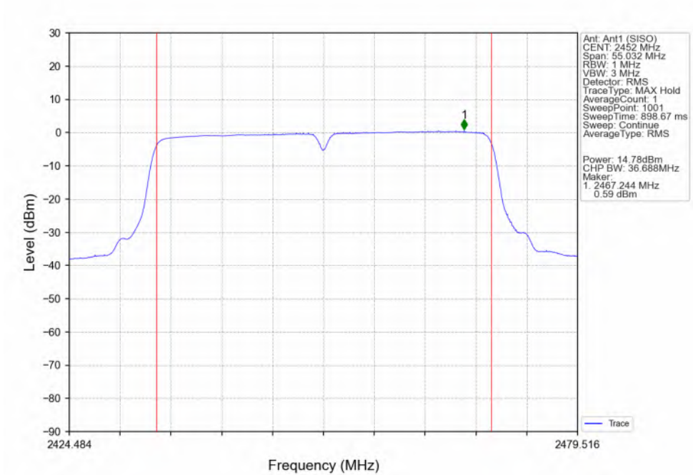
802.11n(HT40)_HCH_2452MHz_Ant1 (SISO)_NTNV
