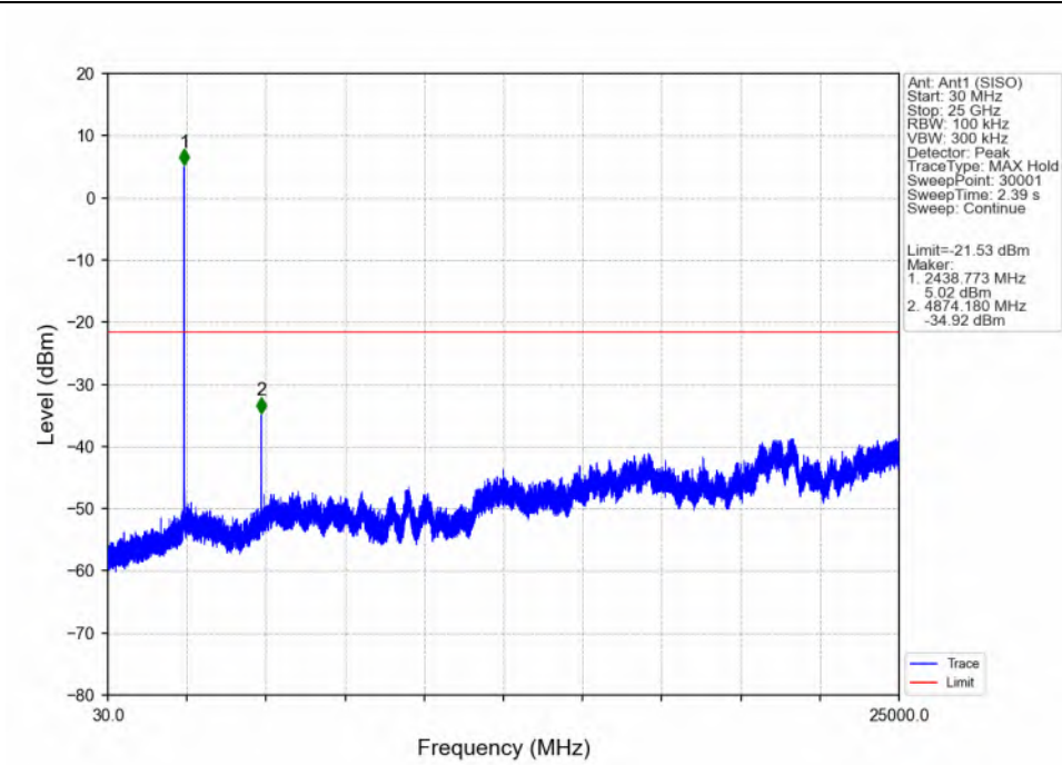
802.11b_MCH_2437MHz_Ant1 (SISO)_NTNV
