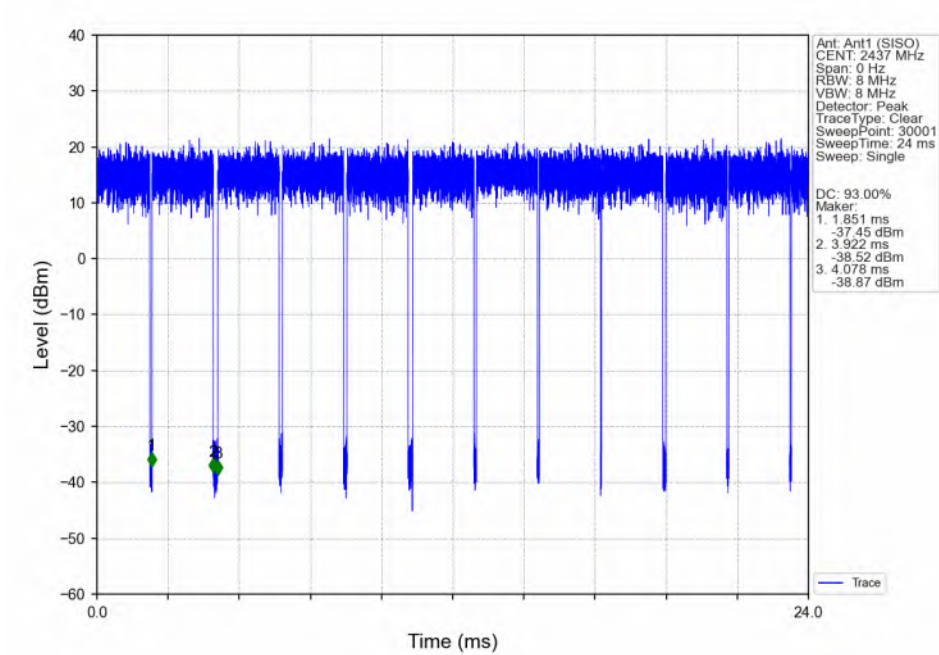
802.11g_MCH_2437MHz_Ant1 (SISO)_NTNV
