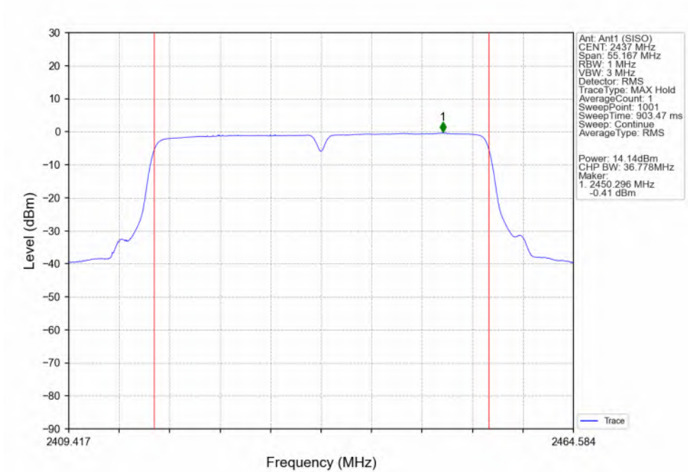
802.11n(HT40)_MCH_2437MHz_Ant1 (SISO)_NTNV
