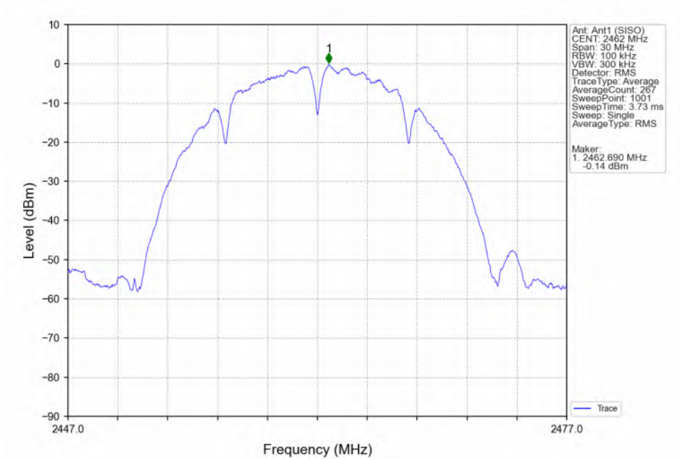
802.11b_HCH_2462MHz_Ant1 (SISO)_NTNV
