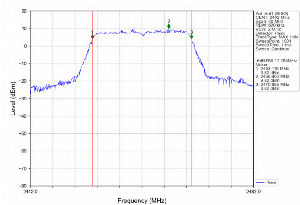
802.11n(HT20)_HCH_2462MHz_Ant1 (SISO)_NTNV
