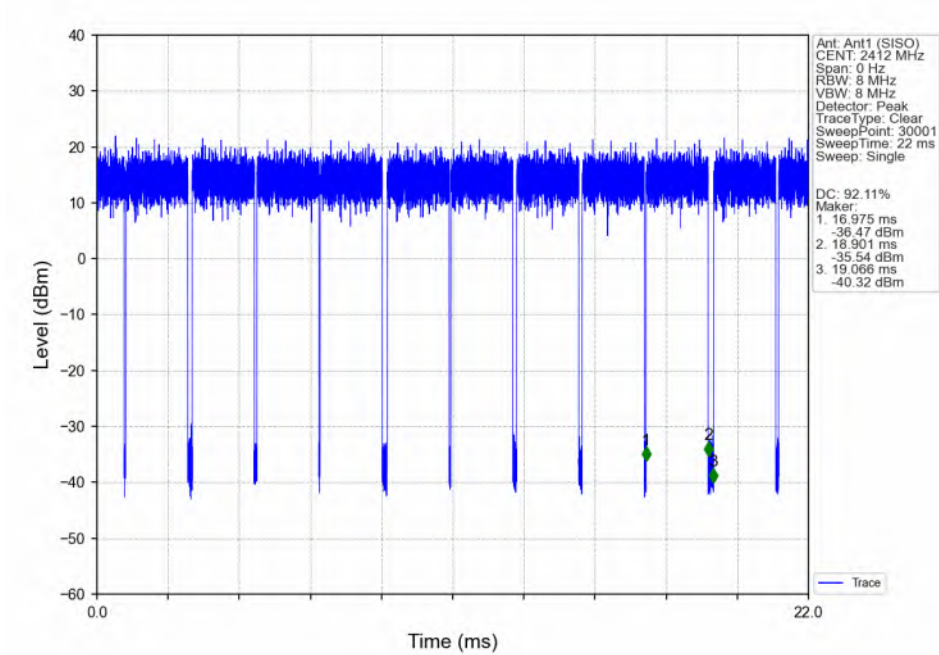
802.11n(HT20)_LCH_2412MHz_Ant1 (SISO)_NTNV
