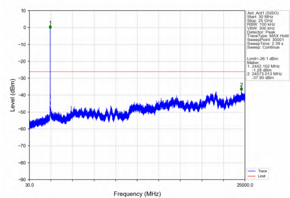
802.11n(HT20)_MCH_2437MHz_Ant1 (SISO)_NTNV
