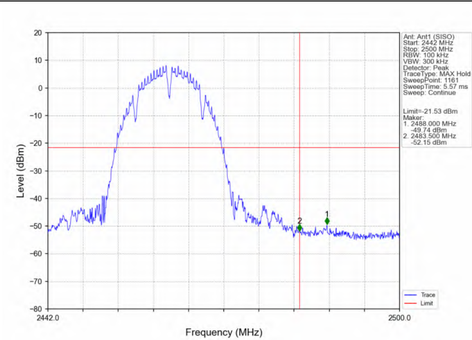
802.11b_HCH_2462MHz_Ant1 (SISO)_NTNV
