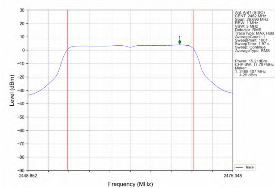
802.11g_HCH_2462MHz_Ant1 (SISO)_NTNV
