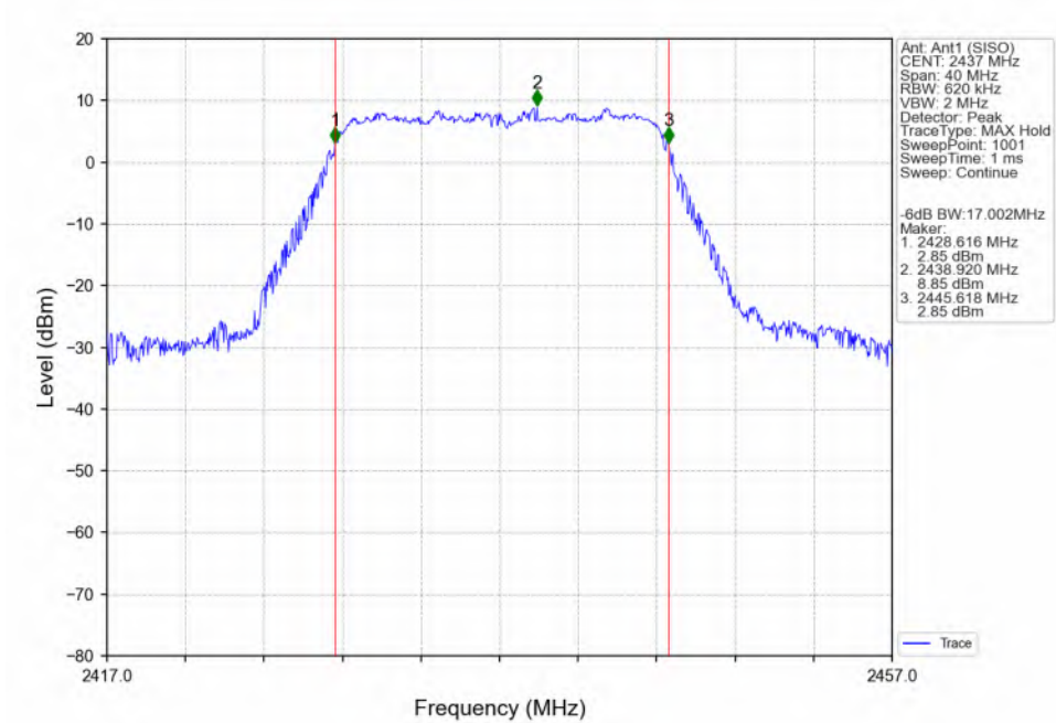
802.11g_MCH_2437MHz_Ant1 (SISO)_NTNV
