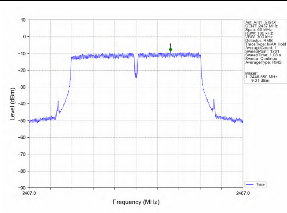
802.11n(HT40)_MCH_2437MHz_Ant1 (SISO)_NTNV
