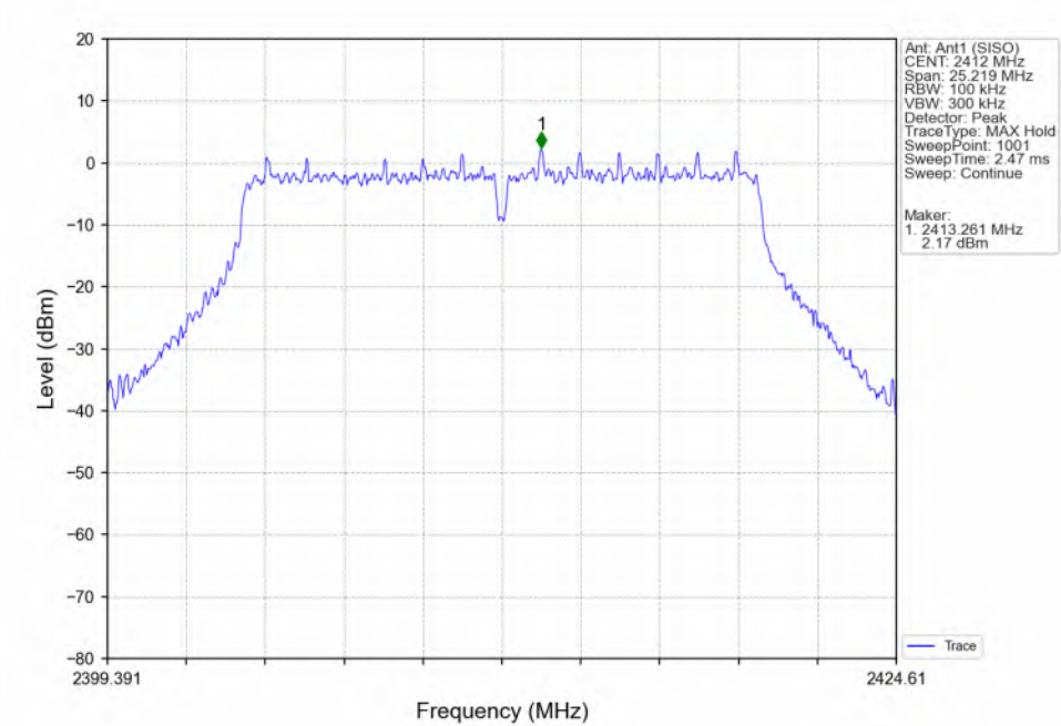
802.11g_LCH_2412MHz_Ant1 (SISO)_NTNV
