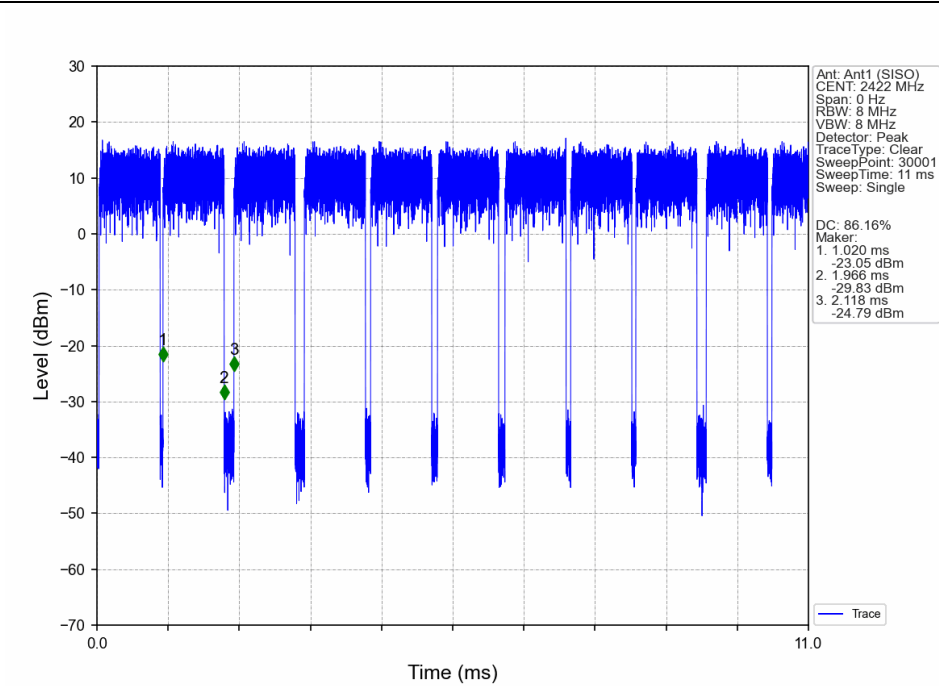
802.11n(HT40)_LCH_2422MHz_Ant1 (SISO)_NTNV
