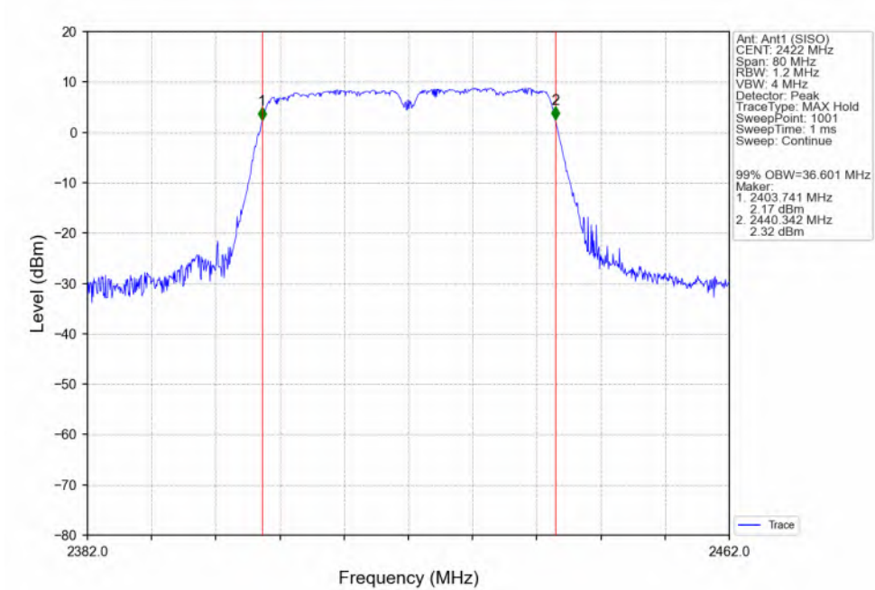
802.11n(HT40)_LCH_2422MHz_Ant1 (SISO)_NTNV
