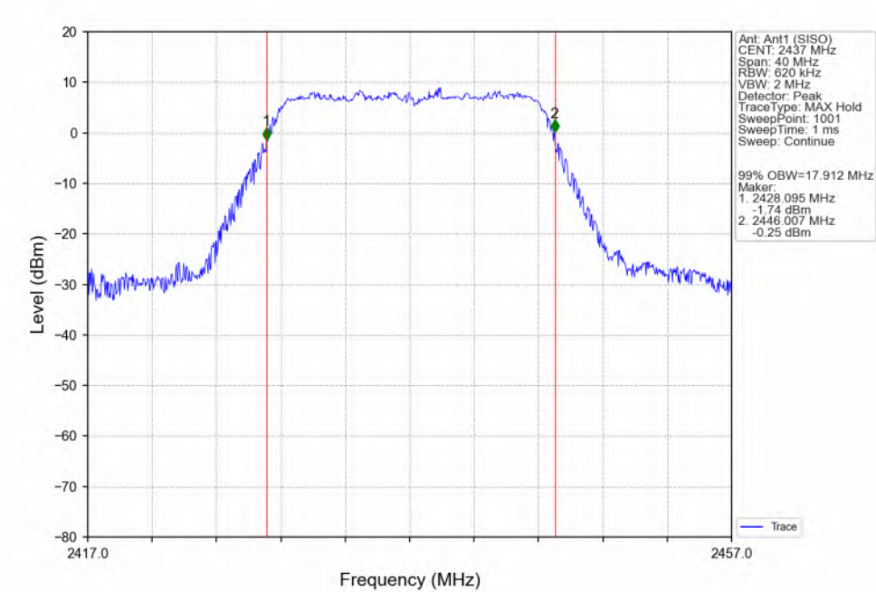
802.11g_MCH_2437MHz_Ant1 (SISO)_NTNV
