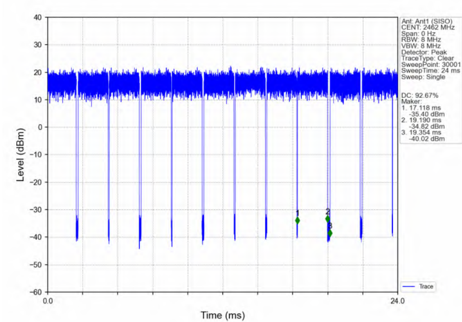
802.11g_HCH_2462MHz_Ant1 (SISO)_NTNV
