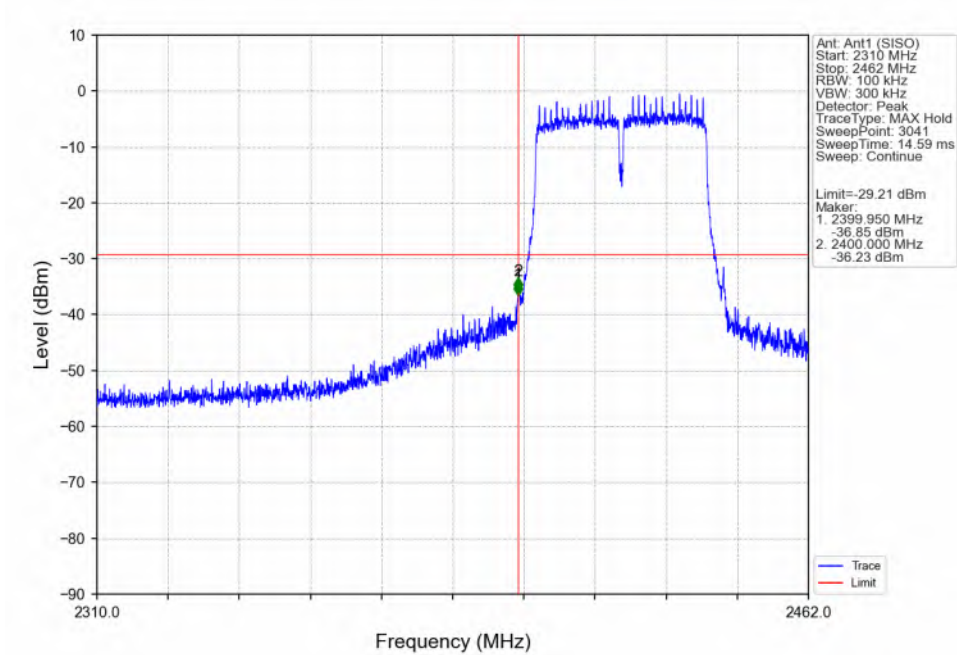
802.11n(HT40)_LCH_2422MHz_Ant1 (SISO)_NTNV
