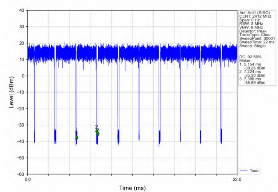
802.11g_LCH_2412MHz_Ant1 (SISO)_NTNV
