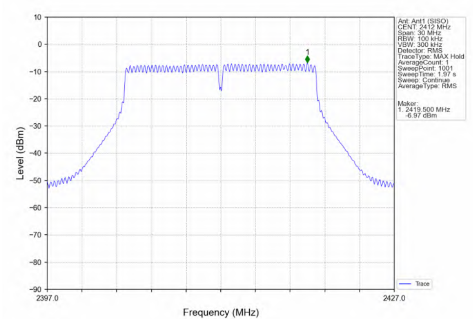
802.11g_LCH_2412MHz_Ant1 (SISO)_NTNV
