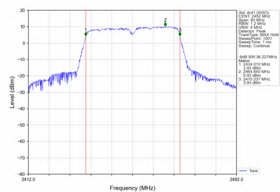
802.11n(HT40)_HCH_2452MHz_Ant1 (SISO)_NTNV
