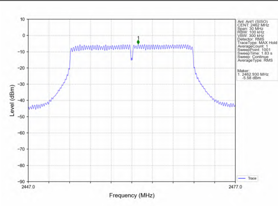
802.11n(HT20)_HCH_2462MHz_Ant1 (SISO)_NTNV
