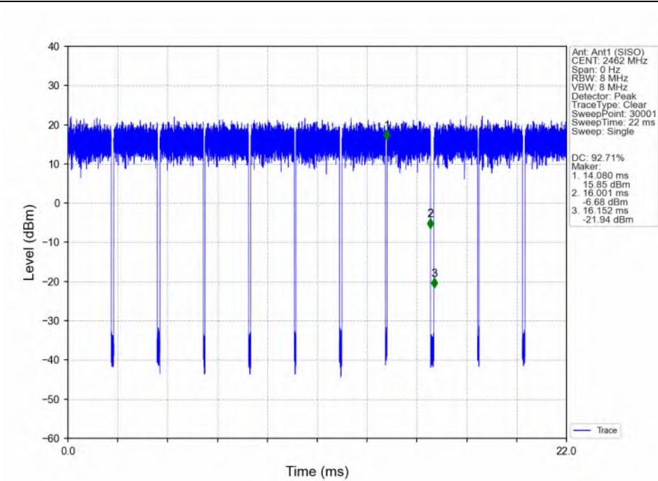
802.11n(HT20)_HCH_2462MHz_Ant1 (SISO)_NTNV
