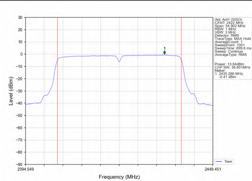
802.11n(HT40)_LCH_2422MHz_Ant1 (SISO)_NTNV
