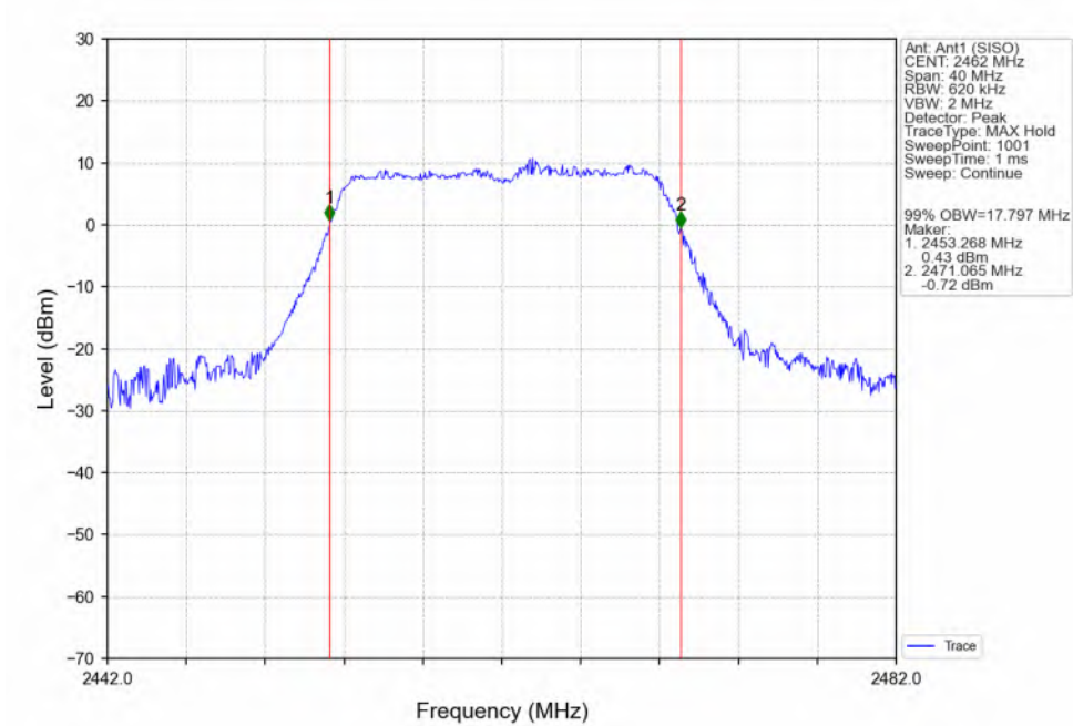
802.11g_HCH_2462MHz_Ant1 (SISO)_NTNV
