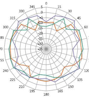
YZ-Plane Gain
