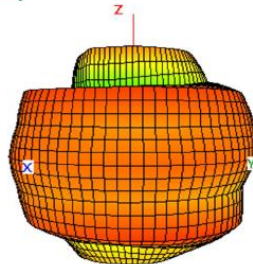
6525 MHz
