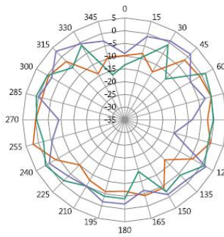
XZ-Plane Gain
