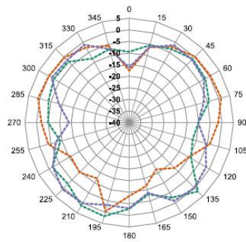
6525 MHz
