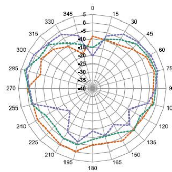
XZ-Plane Gain
