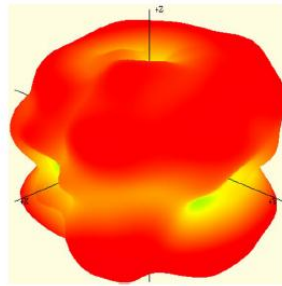
6525 MHz
