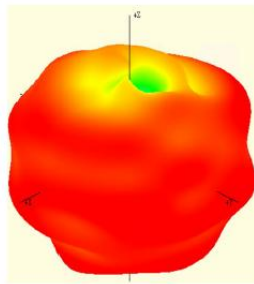
2450 MHz
