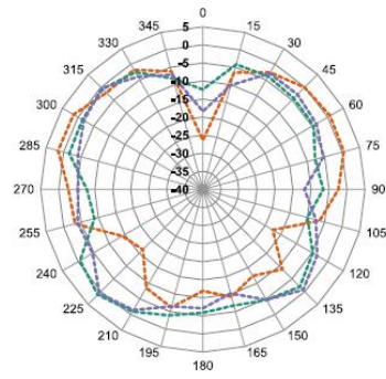
5925 MHz
