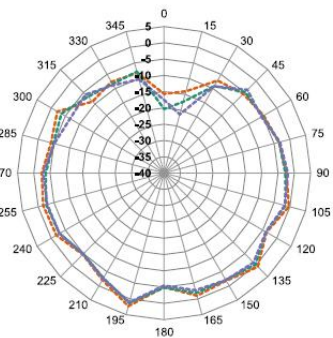
YZ-Plane Gain
