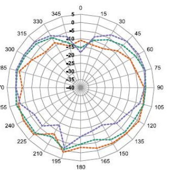
YZ-Plane Gain
