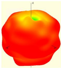
2400 MHz
