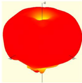
5925 MHz
