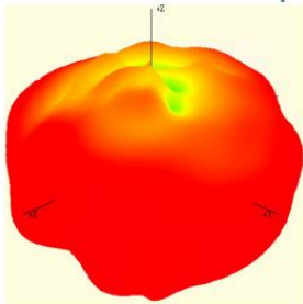
5150 MHz
