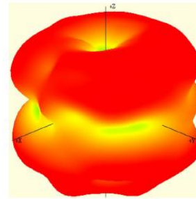
7125 MHz
