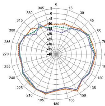
XZ-Plane Gain
