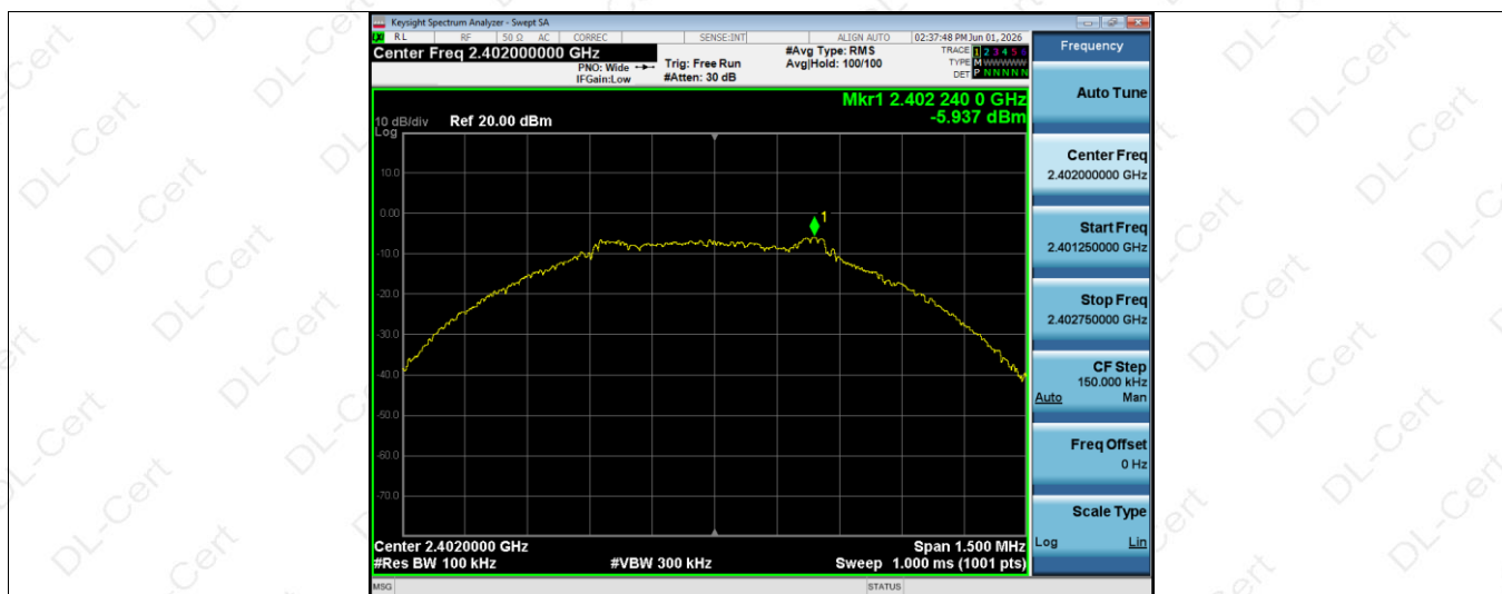
Tx. Spurious NVNT BLE 1M 2402MHz Ant1 Ref
