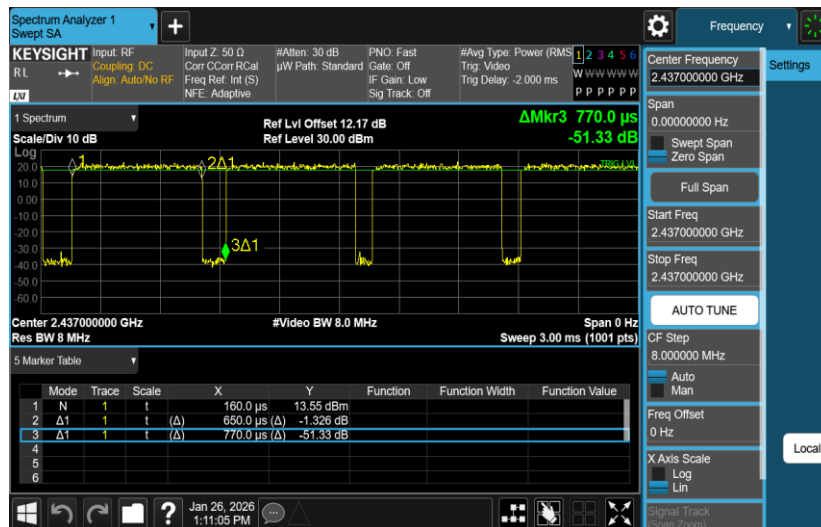
NTNV-11N40MIMO-Ant2-2437
