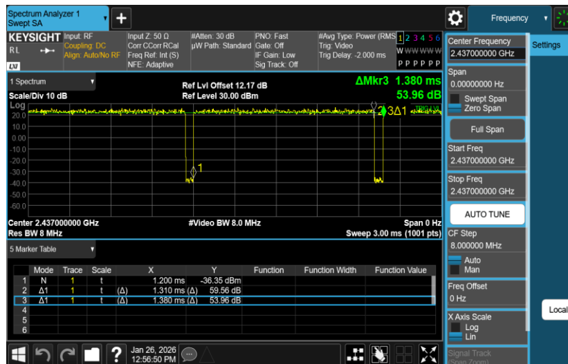
NTNV-11N20MIMO-Ant2-2437
