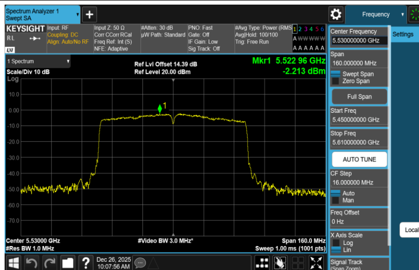
11AC80SISO-Ant2-5530-PASS
