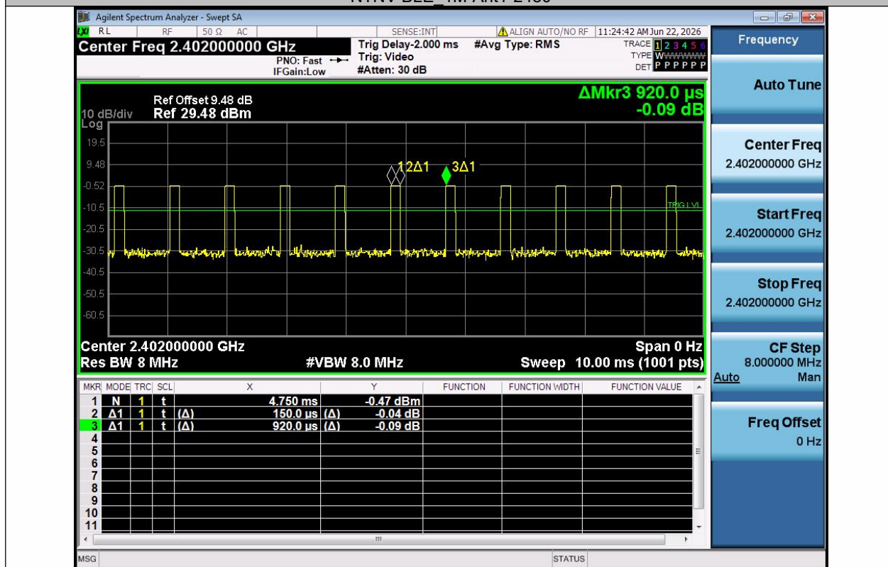
NTNV-BLE_2M-Ant1-2402
