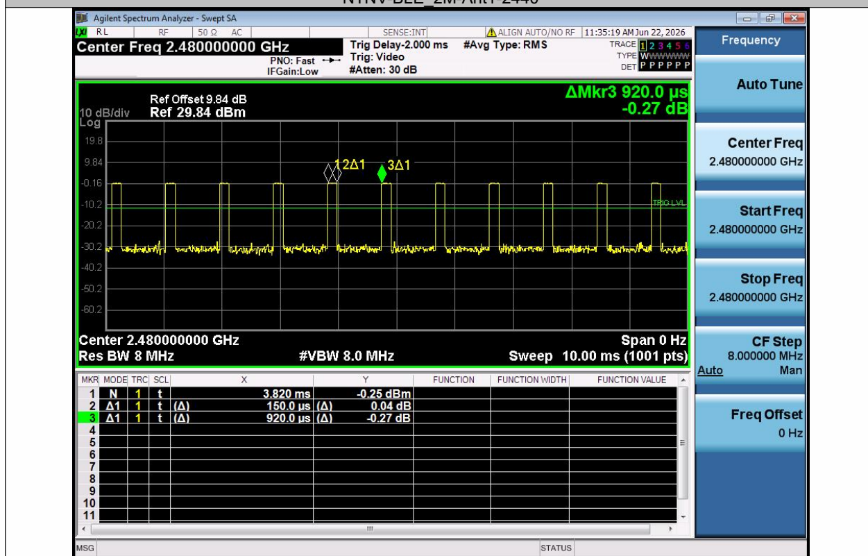
NTNV-BLE_2M-Ant1-2480
