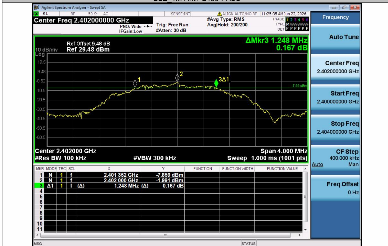
BLE 2M-Ant1-2402-PASS
