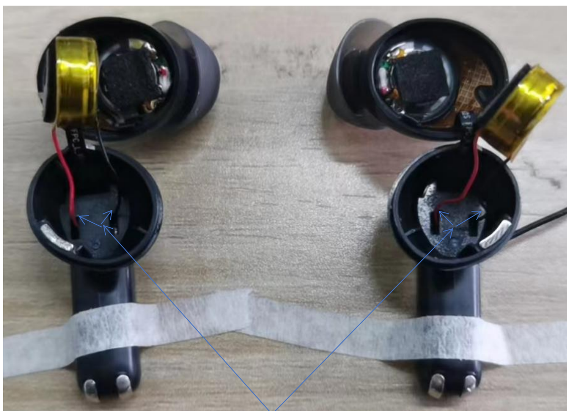
电池红黑线如图穿孔，拉出 主板下多余的电池线到前腔
