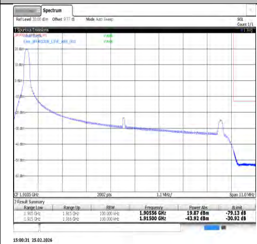
Band25-10MHz-QPSK-26640-50RB#0-PASS
