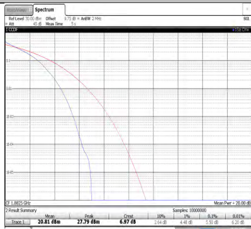
Band25-1.4MHz-QPSK-26365-6RB#0-PASS
