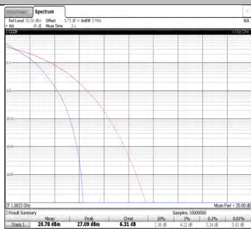
Band25-5MHz-QPSK-26365-25RB#0-PASS
