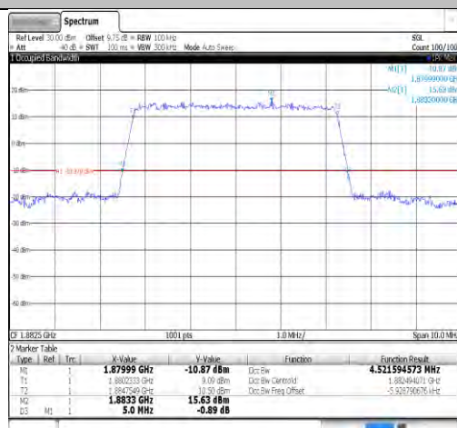
Band25-5MHz-QPSK-26365-25RB#0-PASS
