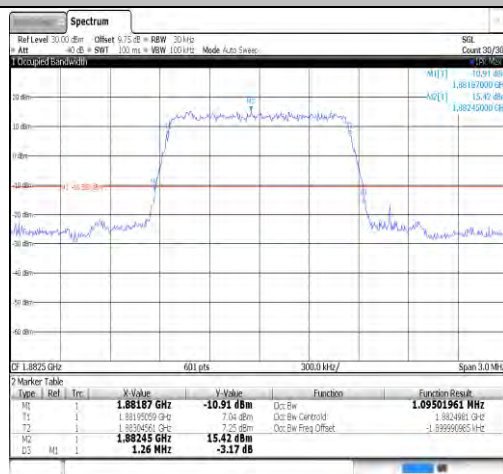
Band25-1.4MHz-QPSK-26365-6RB#0-PASS
