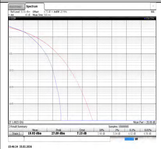
Band25-20MHz-16QAM-26365-100RB#0-PASS
