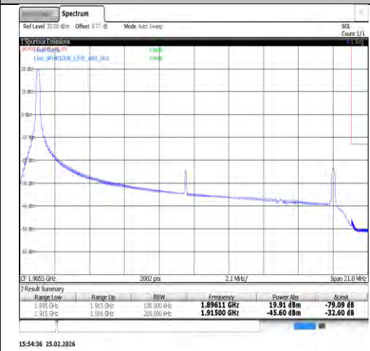
Band25-20MHz-QPSK-26590-100RB#0-PASS
