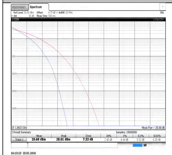
Band25-20MHz-QPSK-26365-100RB#0-PASS
