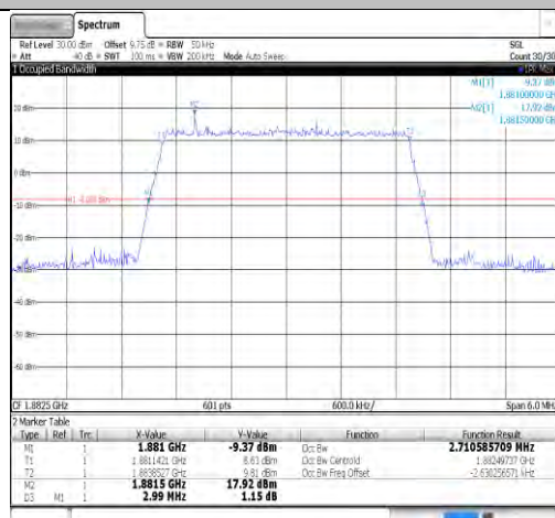
Band25-3MHz-QPSK-26365-15RB#0-PASS
