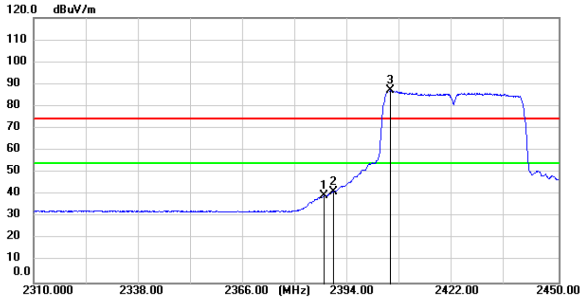
11n(HT40)_TX_CH_03_Horizontal_Average
