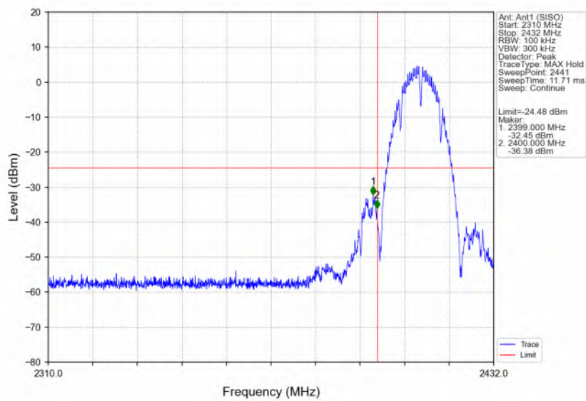
802.11b_LCH_2412MHz_Ant1 (SISO)_NTNV
