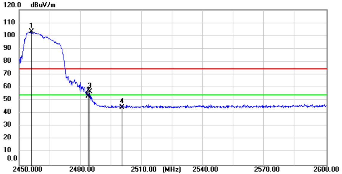
11n(HT20)_TX_CH_11_Horizontal_Peak
