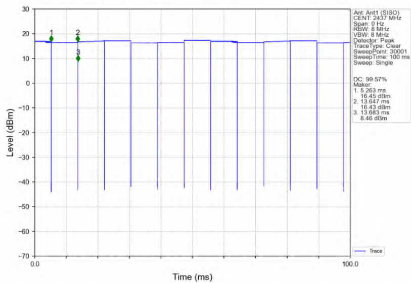
802.11b_MCH_2437MHz_Ant1 (SISO)_NTNV
