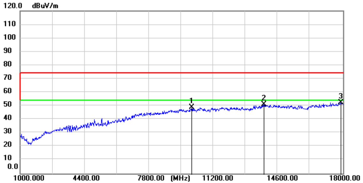
11n(HT20)_TX_CH_11_Vertical
