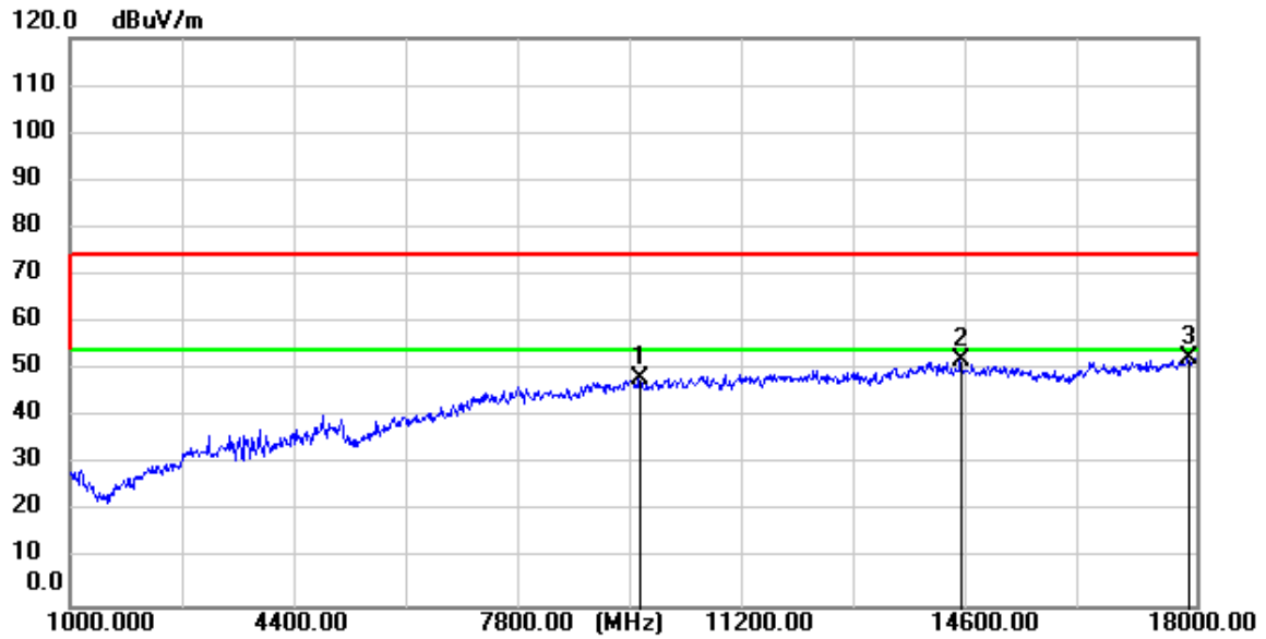
11b_TX_CH_01_Vertical
