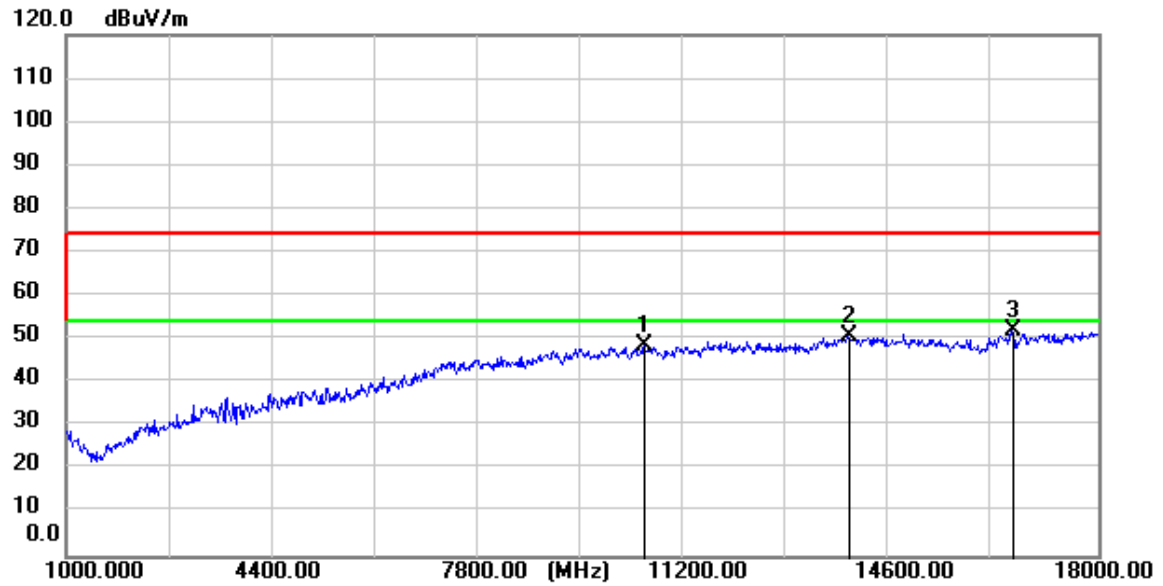
11n(HT40)_TX_CH_09_Vertical
