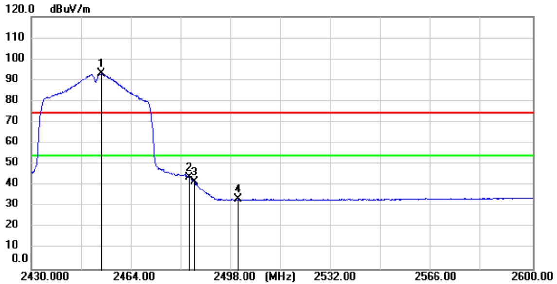
11n(HT40)_TX_CH_09_Horizontal_Average
