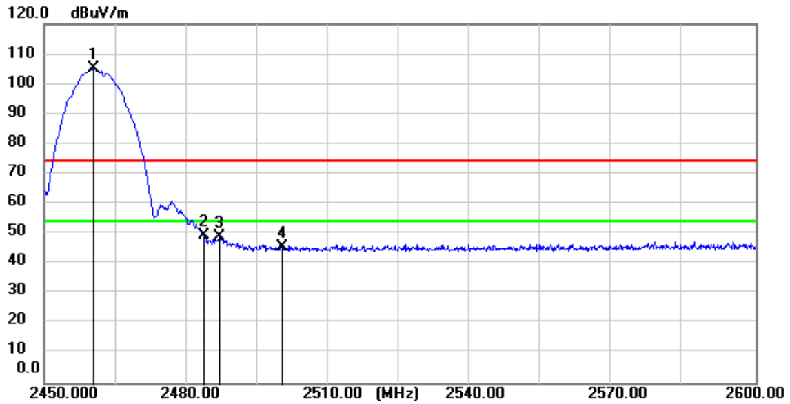
11b_TX_CH_11_Horizontal_Peak
