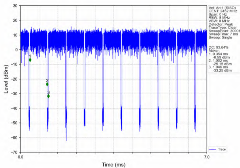
802.11n(HT40)_HCH_2452MHz_Ant1 (SISO)_NTNV
