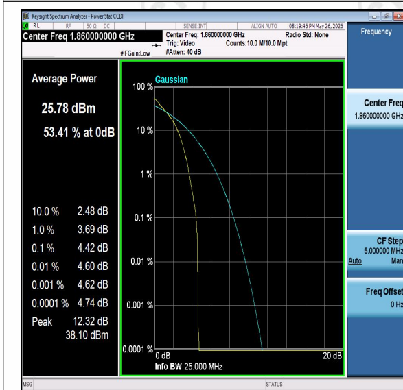
Band2-20MHz-QPSK-18700-PASS
