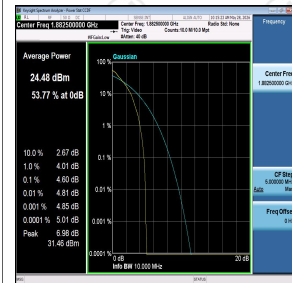
Band25-10MHz-QPSK-26365-PASS
