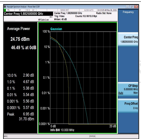
Band25-10MHz-16QAM-26365-PASS
