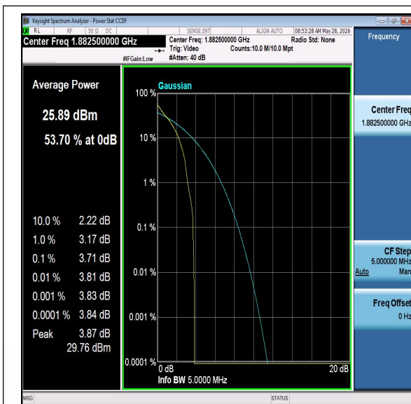
Band25-5MHz-QPSK-26365-PASS
