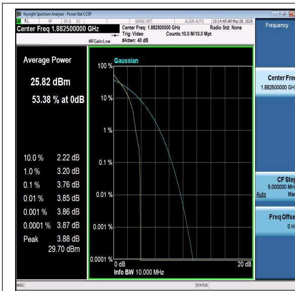
Band25-10MHz-QPSK-26365-PASS
