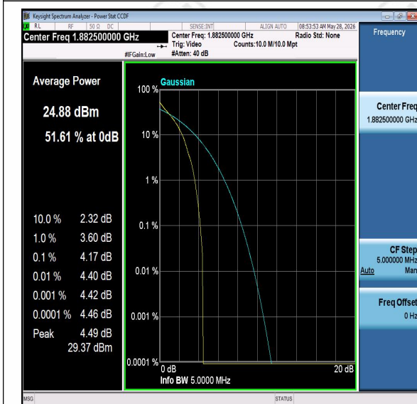
Band25-5MHz-QPSK-26365-PASS
