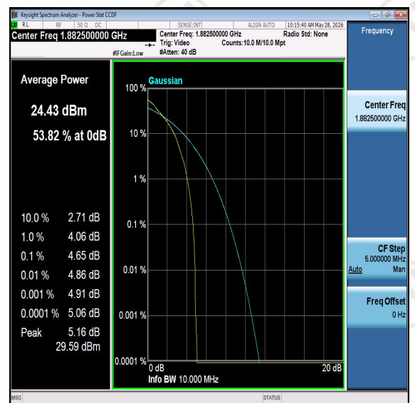
Band25-10MHz-16QAM-26365-PASS
