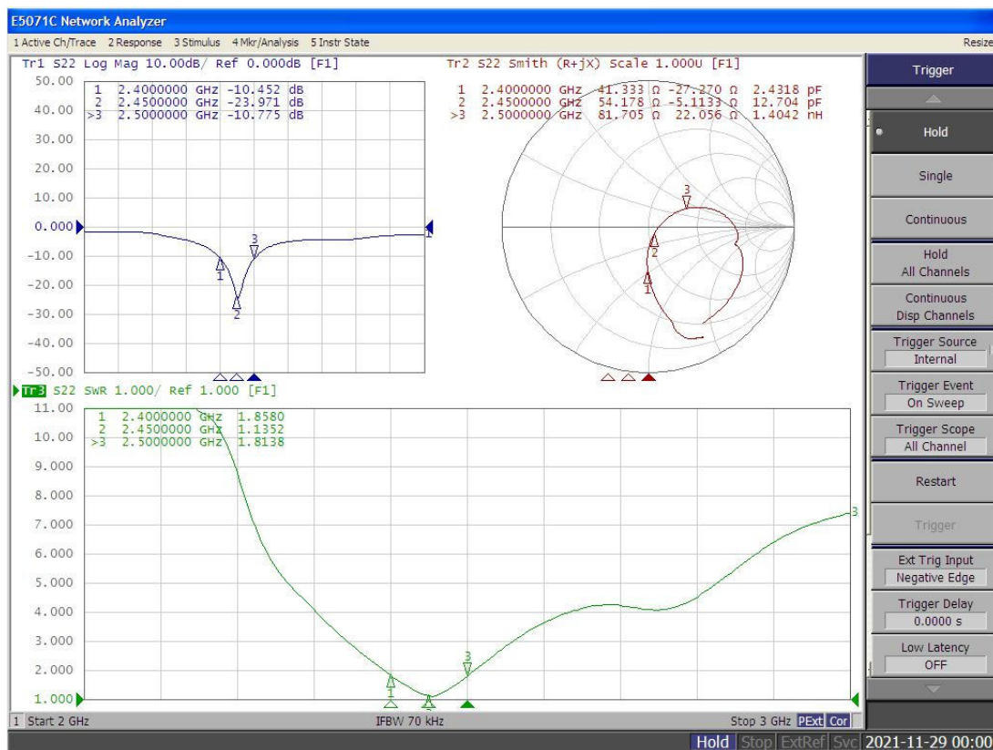
Antenna S parameters
