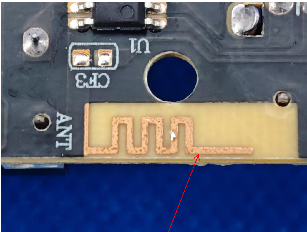
PCB ANT
